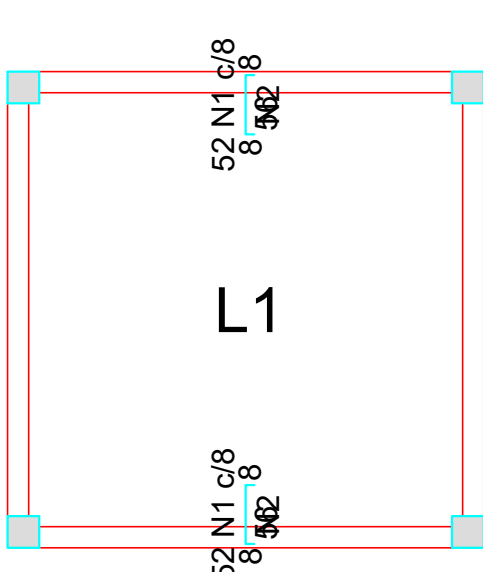
Armação negativa das lajes do pavimento terreo (Eixo Y) escala 1:50
