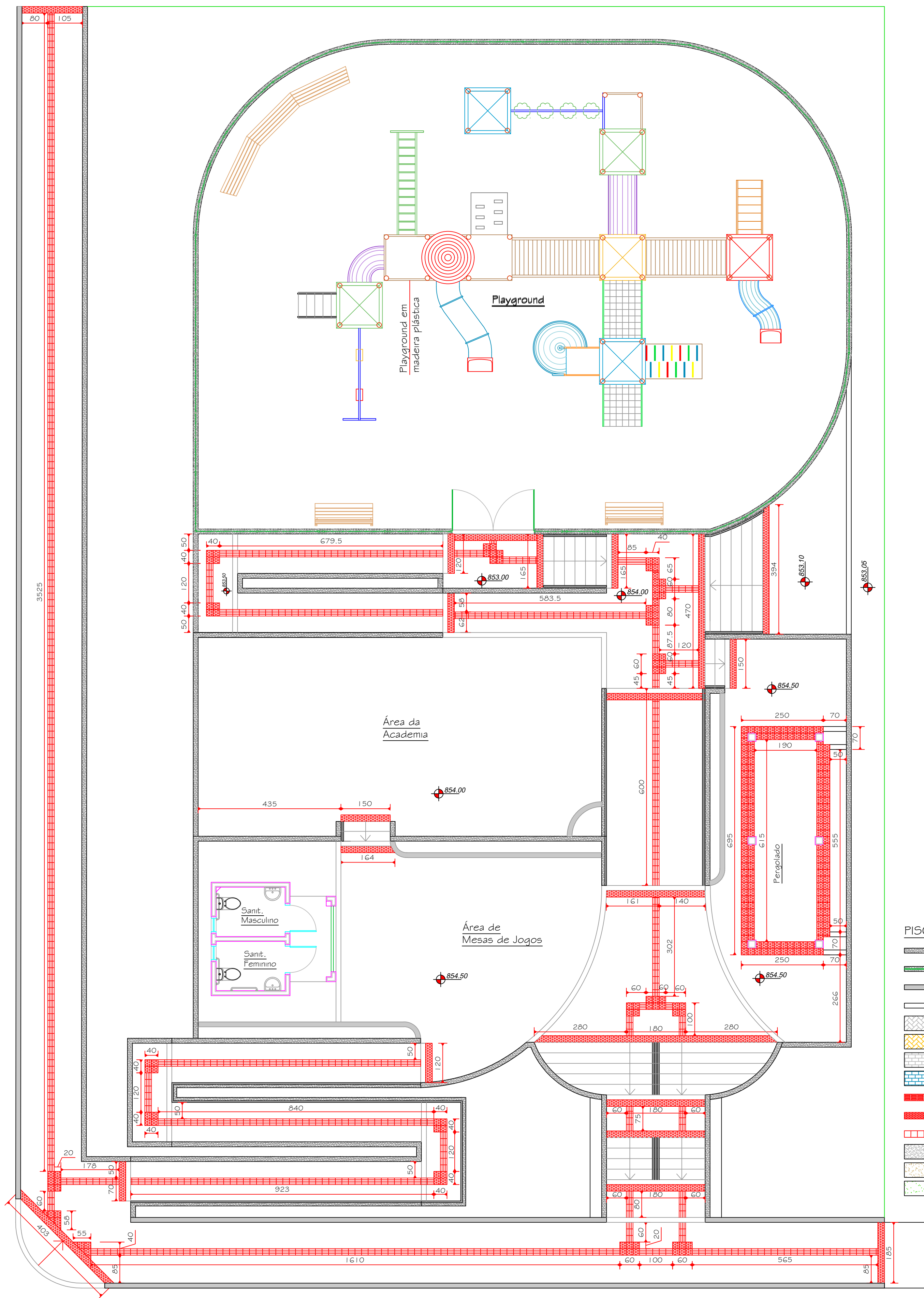
PLANTA DE ACESSIBILIDADE Escala 1/75 Área Total: 1.020,16m²
