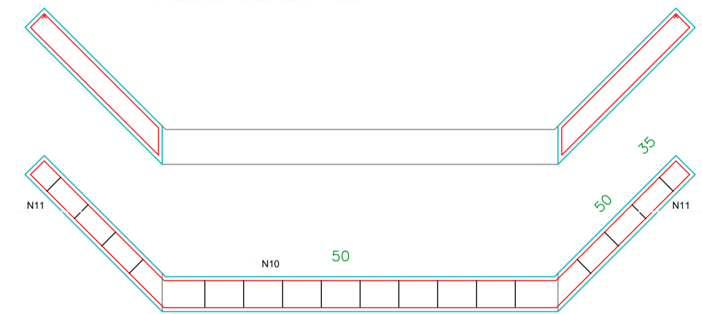
Armaduras horizontais - Alas
