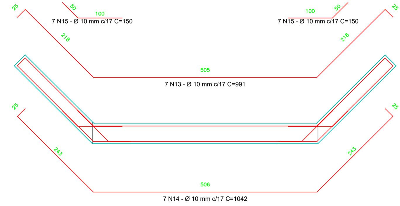
Armaduras horizontais - Corrimão e Alas
