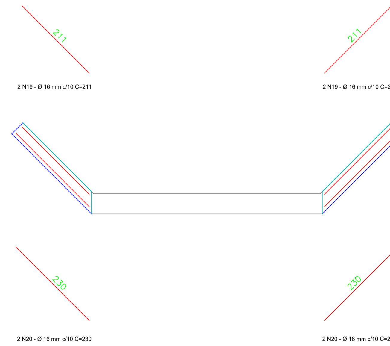
DETALHE REFORÇO DO TOPO DAS ALAS
