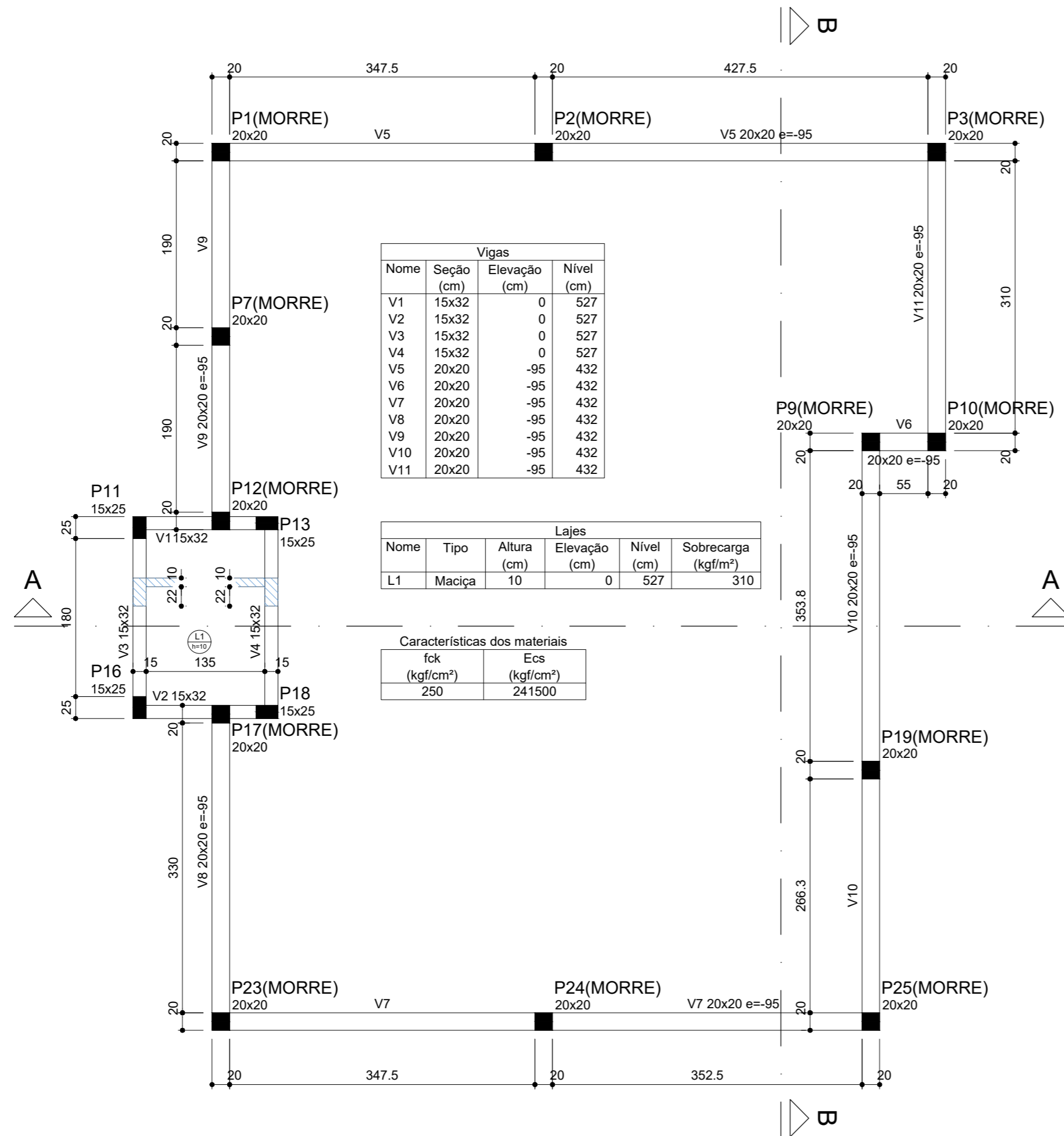
Forma do pavimento RESERVATÓRIO (Nível 527) escala 1:50
