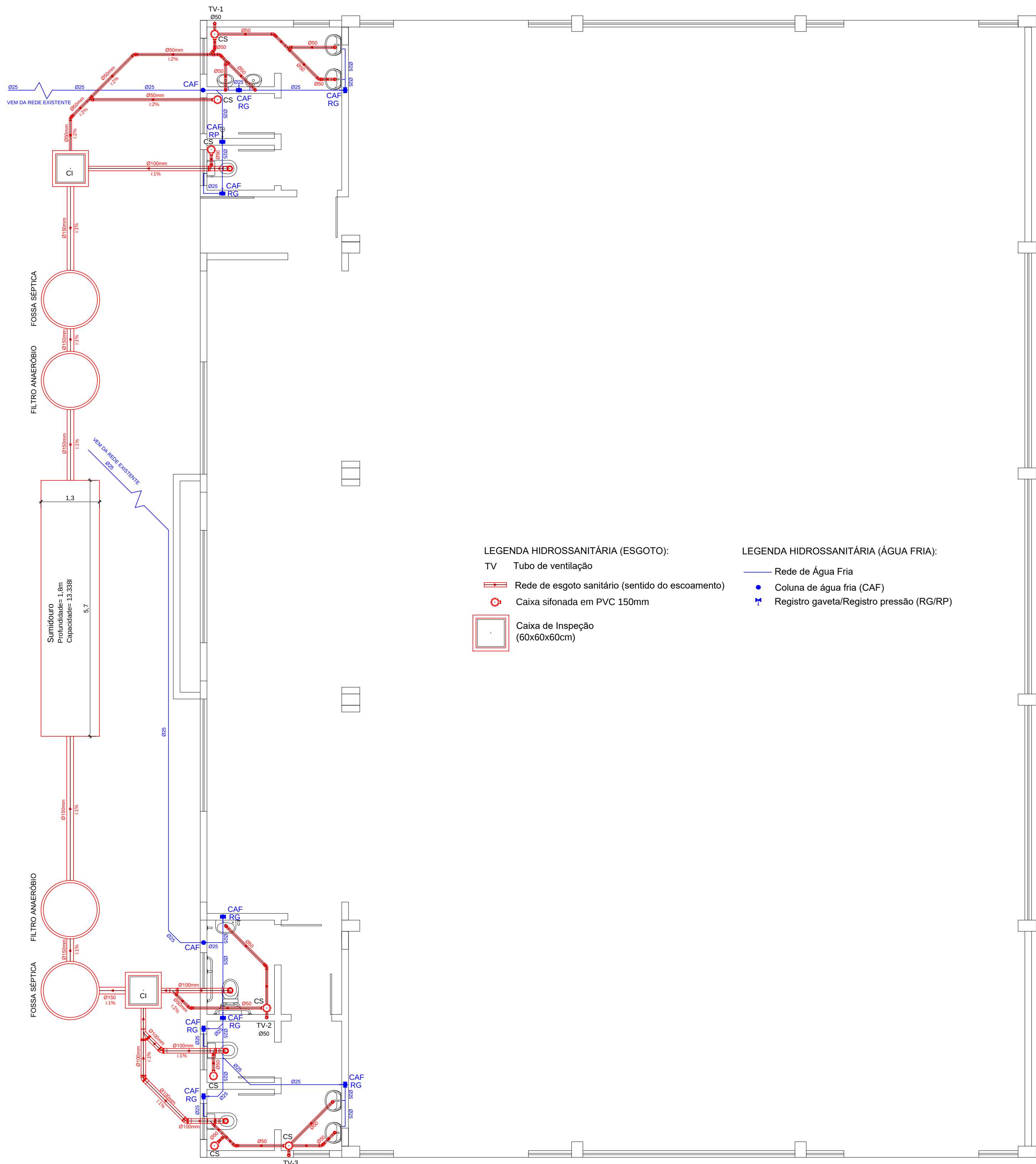
INSTALAÇÕES HIDROSSANITÁRIAS Escala 1/60
