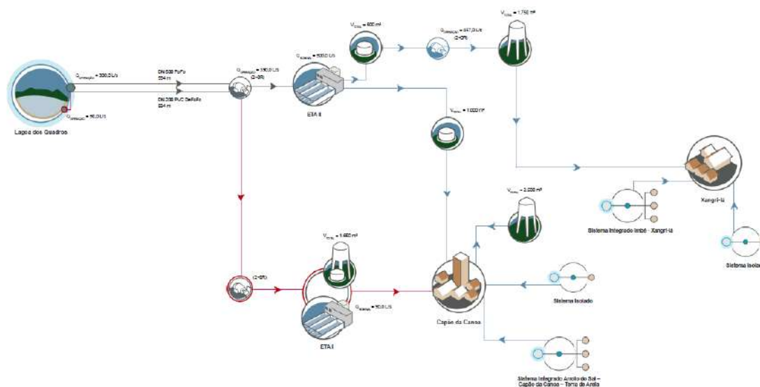
Figura 84 – Croqui - Sistema Integrado Capão da Canoa – Xangri-lá | RS.
