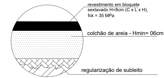
DETALHE 02 - CORTE CAMADA BLOQUETE, PARALELEPIPEDO E INTERTRAVADO SEM ESCALA
