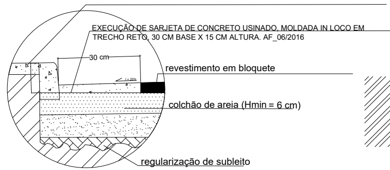
DETALHE 01 - MEIO FIO E SARJETA - PISO BLOQUETE SEM ESCALA
