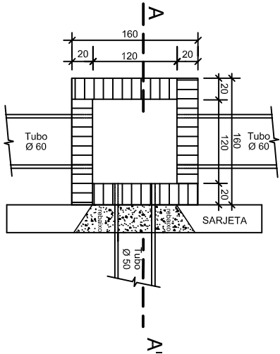
PLANTA BAIXA - BOCA DE LOBO (1,60 x 1,60m) S/Escala
