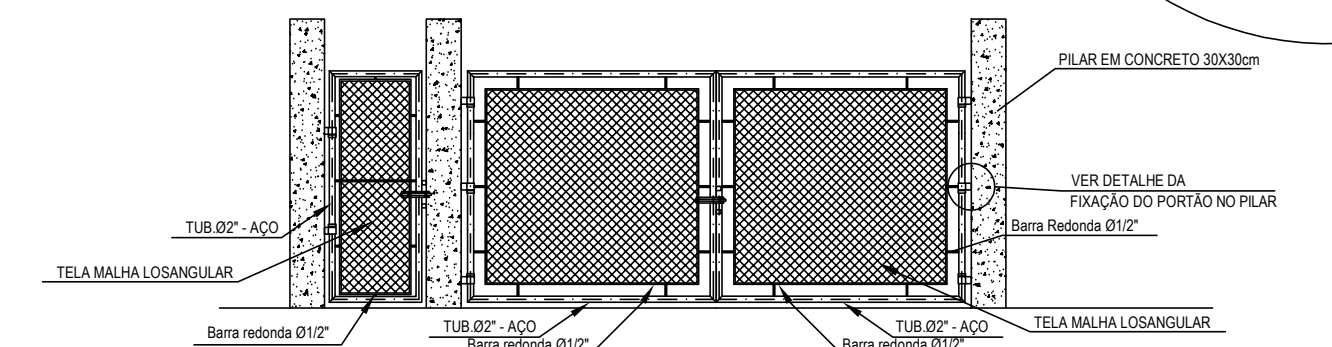
DETALHE 2 - PORTÃO DE ACESSO
