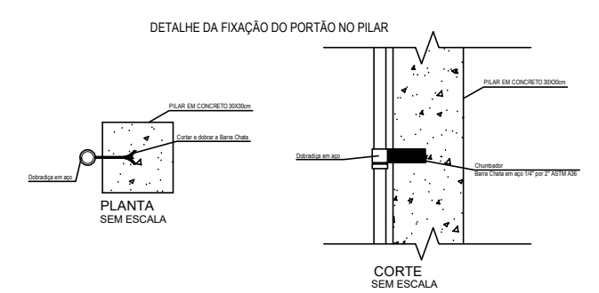
DETALHE 2 - PORTÃO DE ACESSO
