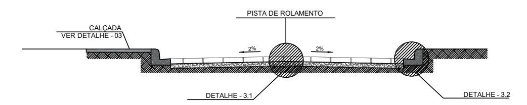
SEÇÃO TRANSVERSAL AA' - PAVIMENTAÇÃO EM BLOCKRET ESC: 1/40
