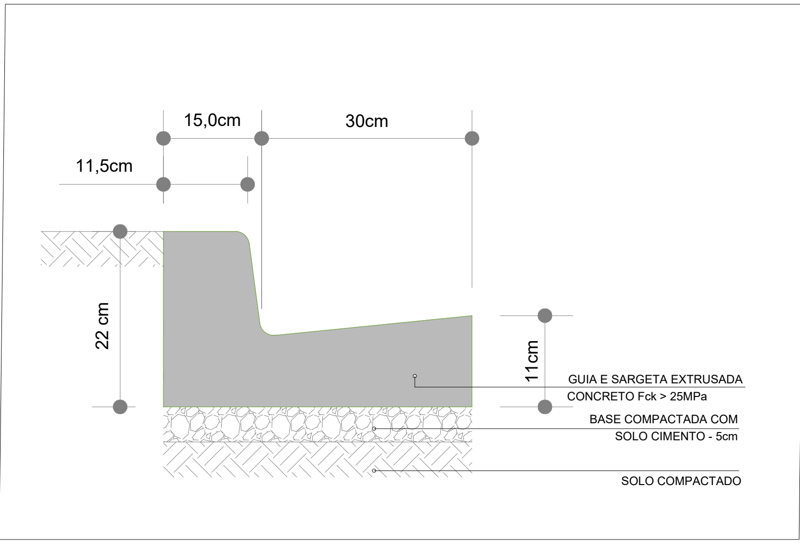
2 DETALHE GUIA E SARJETA SEM ESCALA
