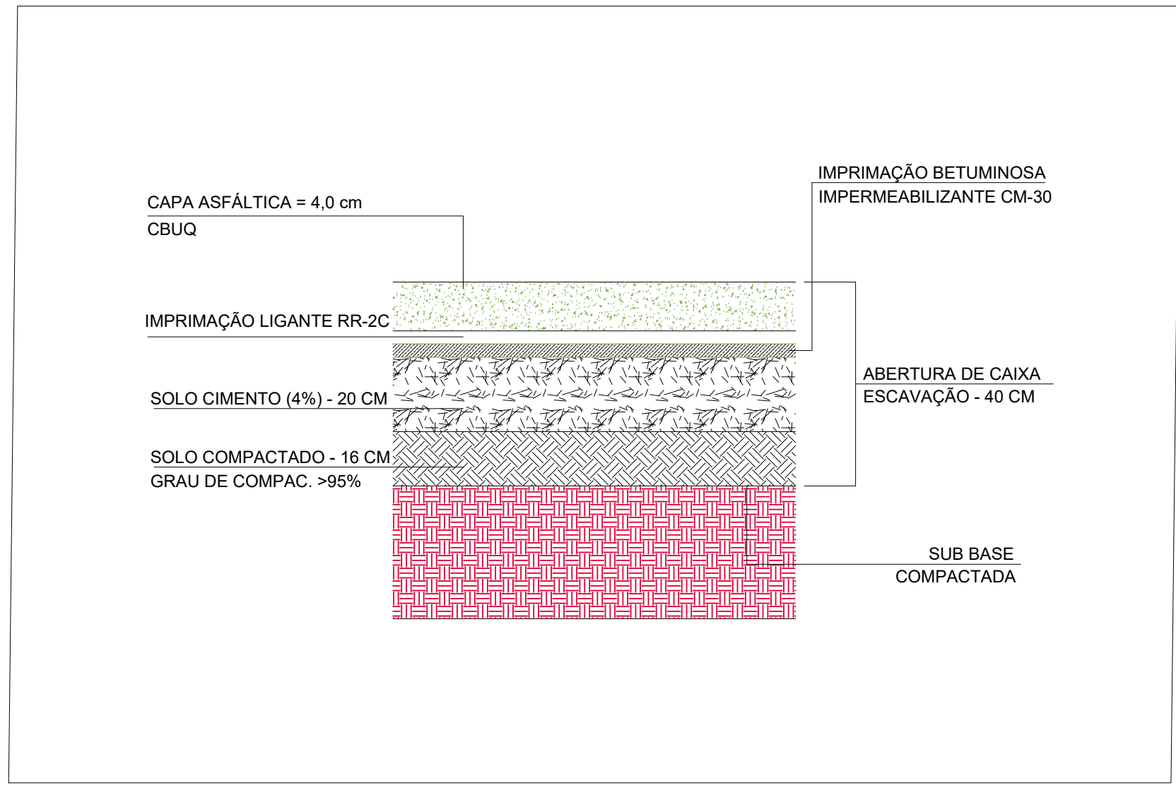
1 DETALHE CAMADAS PAVIMENTAÇÃO SEM ESCALA
