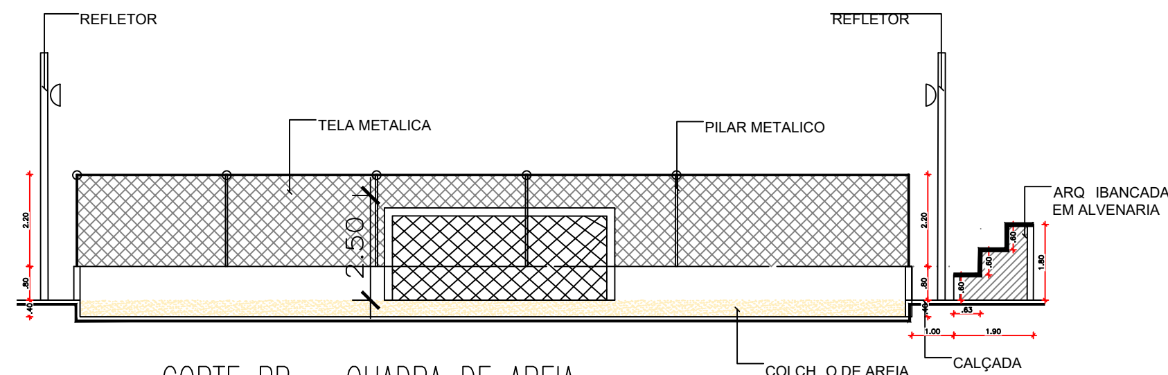
CORTE BB – QUADRA DE AREIA ESCALA 1/250
