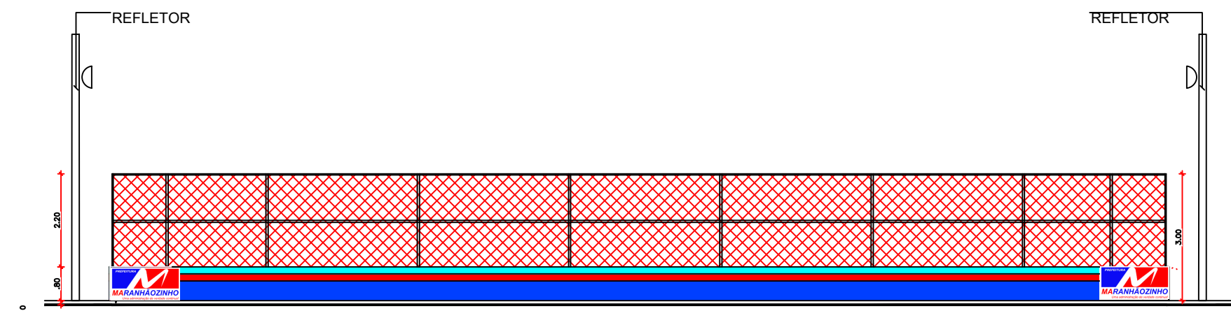
CORTE BB – QUADRA DE AREIA ESCALA 1/250
