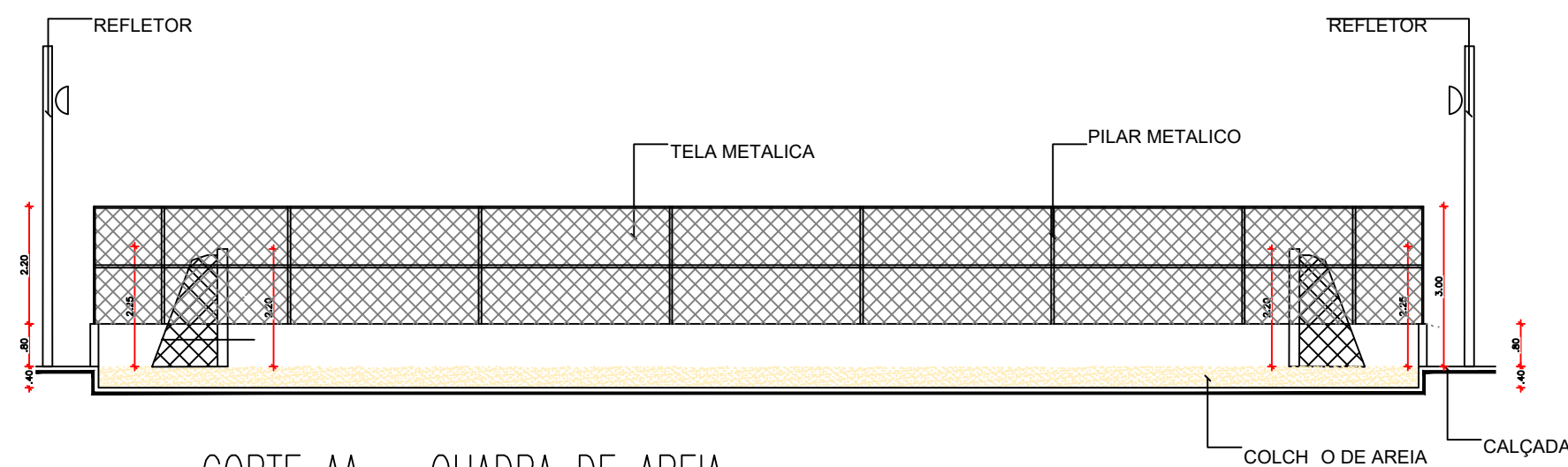
CORTE AA – QUADRA DE AREIA ESCALA 1/250
