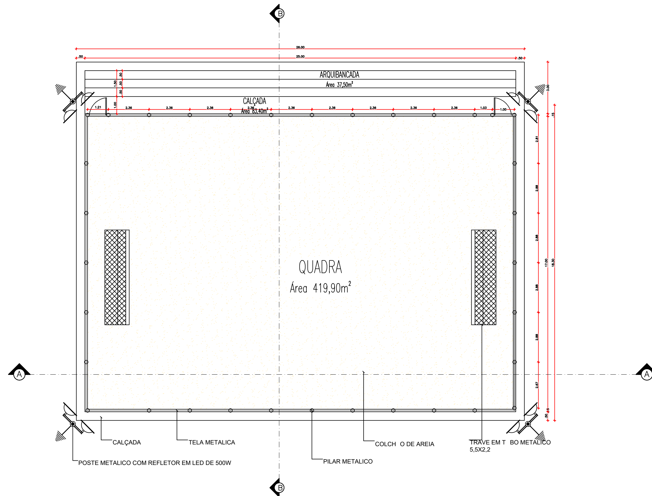
PLANTA BAIXA – QUADRA DE AREIA ESCALA 1/250
