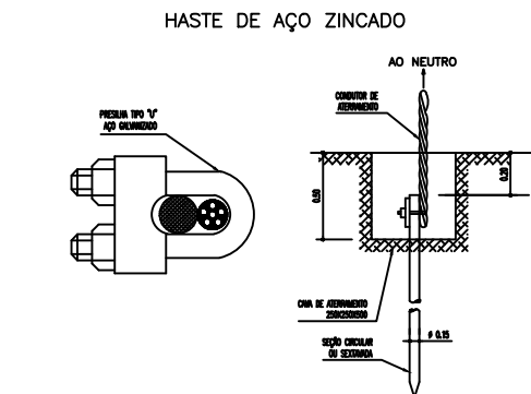
DETALHE DA CONEXÃO DO CABO COM A HASTE DE ATERRAMENTO EM CADA POSTE SEM ESCALA
