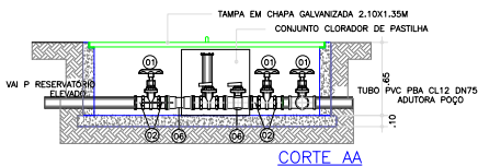
CORTE AA
