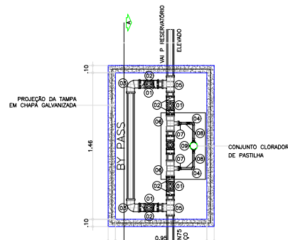
PLANTA BAIXA
