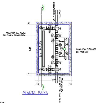
DET.-03 DETALHE DA CAIXA DE INSPEÇÃO DO CLORADOR SEM ESCALA
