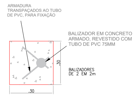
DETALHE 01 - BALIZADOR 1 : 50
