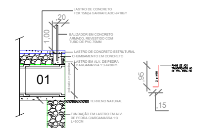
DETALHE 02 - BALIZADOR 1 : 50
