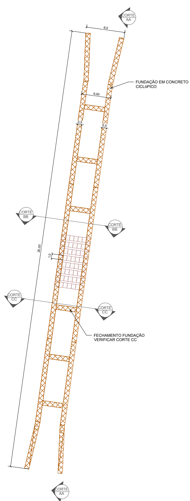
FUNDAÇÃO - PASSAGEM MOLHADA 1 : 250
