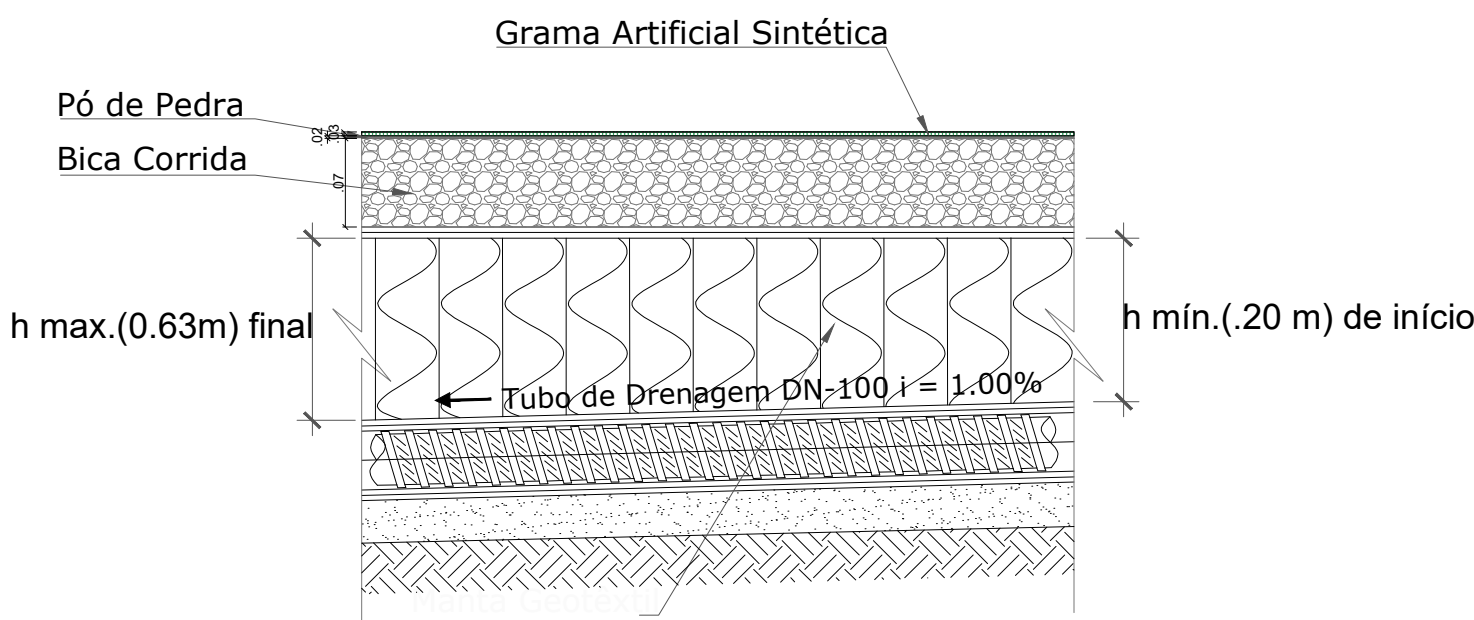
DETALHE DA ALTURA MIN E MAX DO TUBO DE DRENAGEM
