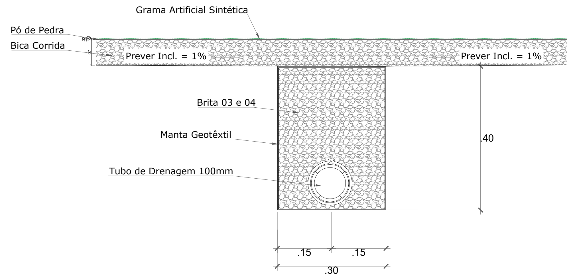
CORTE DETALHE VALA DRENAGEM
