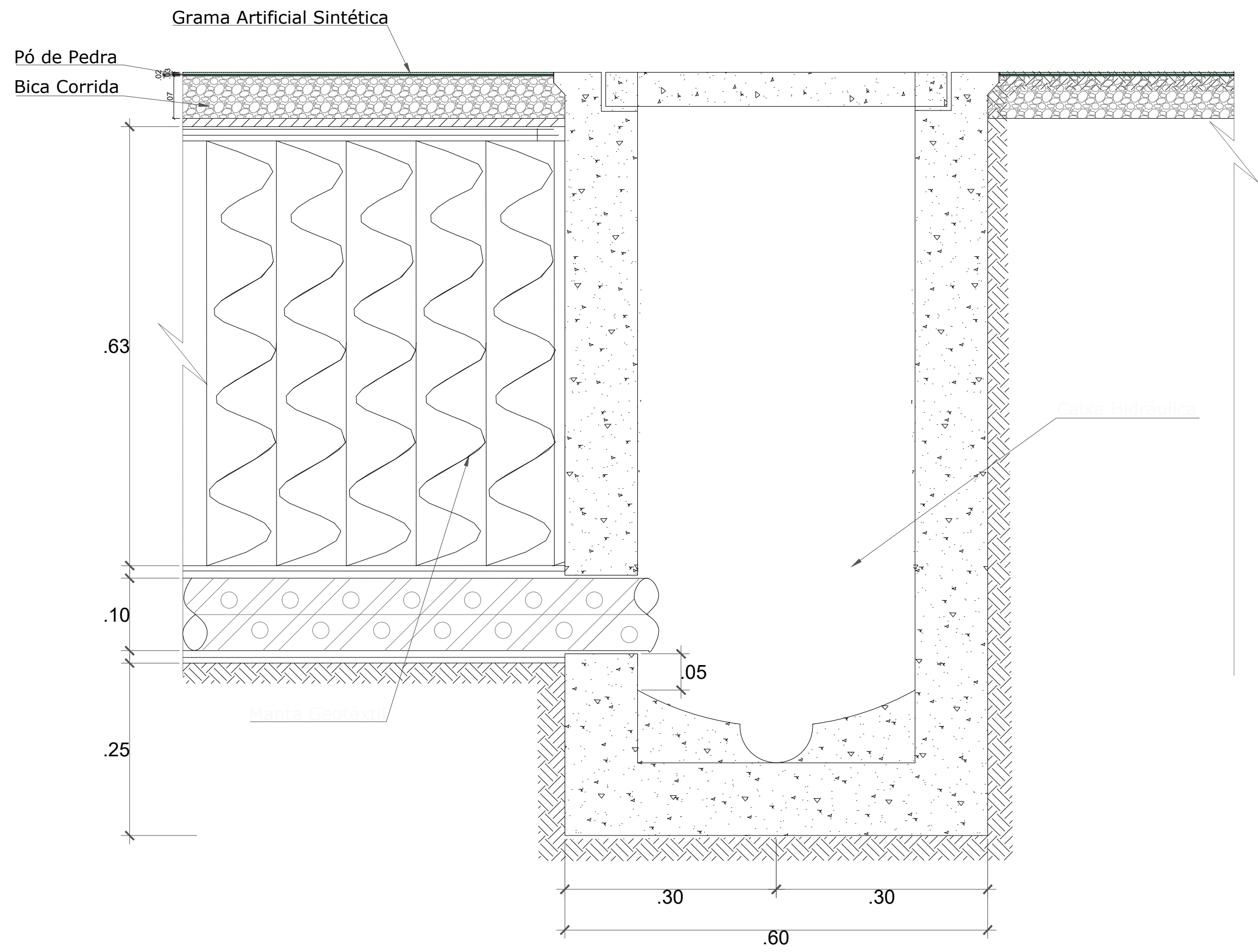
DETALHE DE CHEGADA DE TUBO FLEXÍVEL (Tubo DN-100) PARA CAIXA HIDRÁULICA
