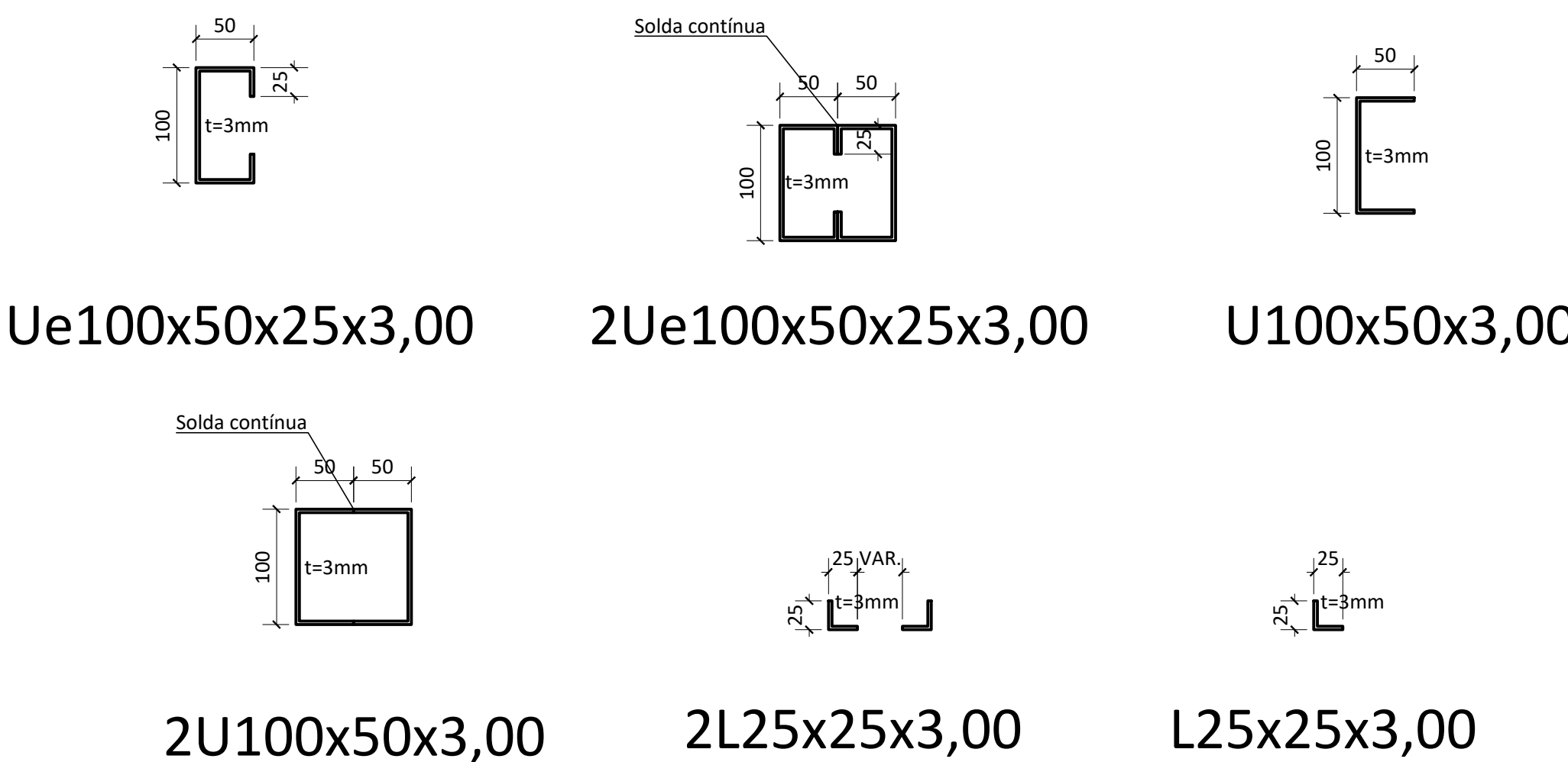
DETALHE DE PERFIS ESTRUTURAIS
