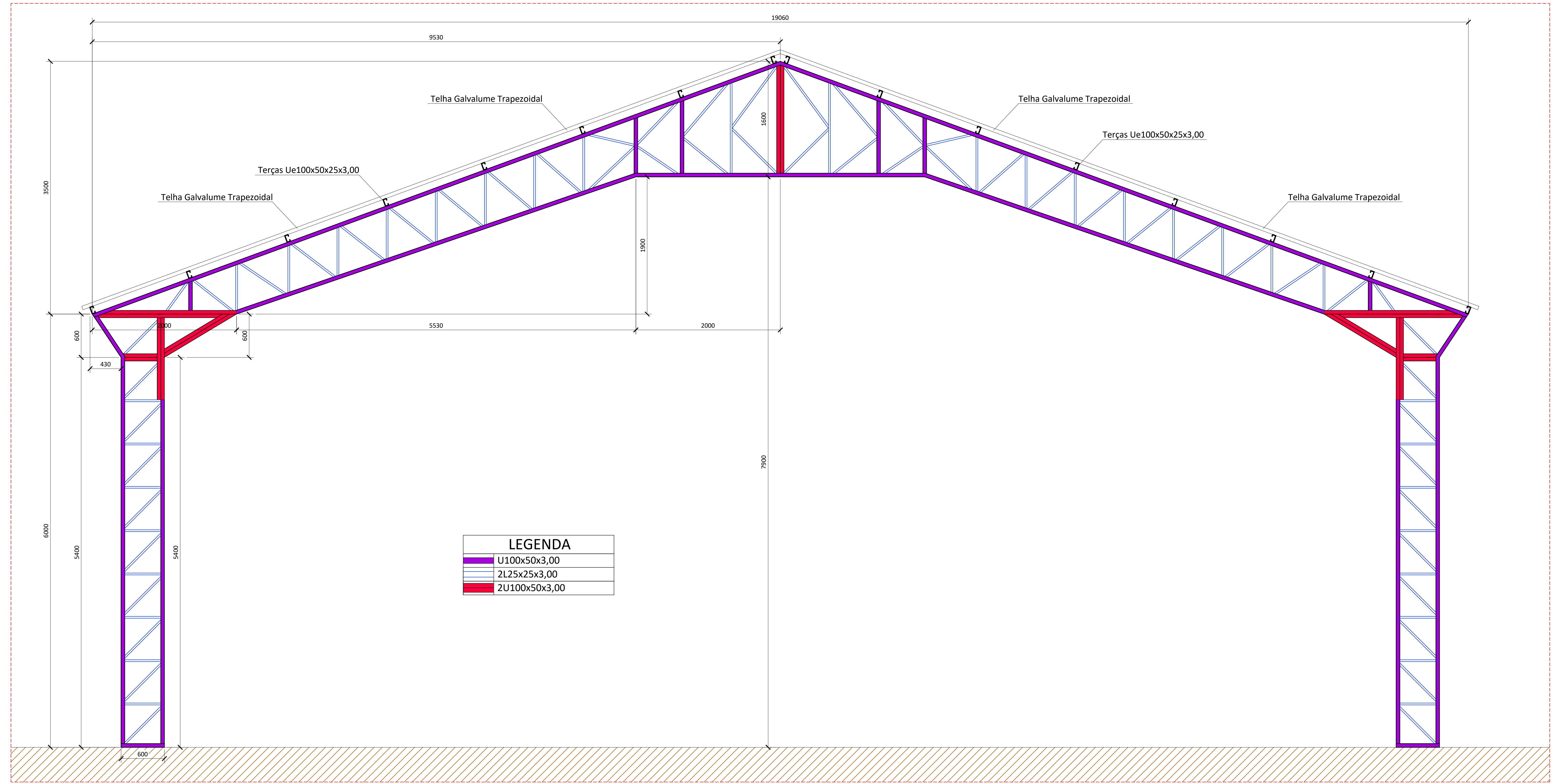
CORTE AA - DETALHE DE TRELIÇA 01 (7x)
