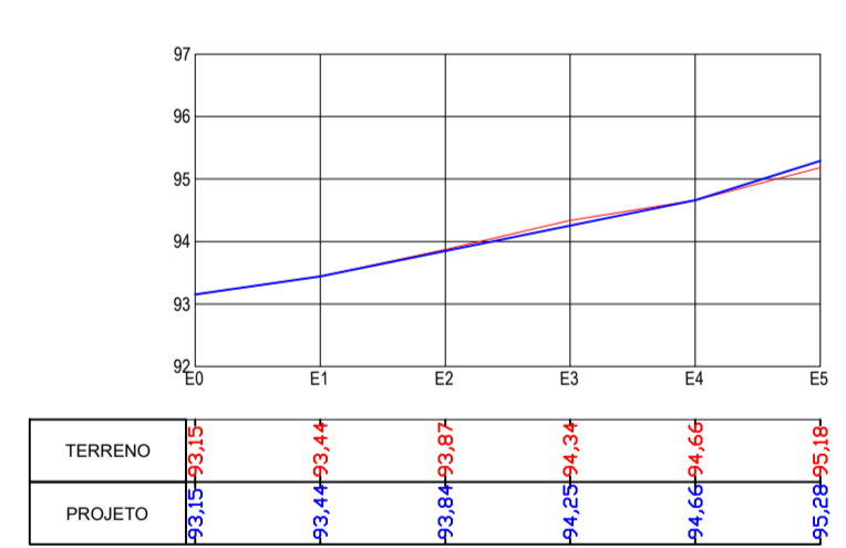
PERFIL RUA 2
