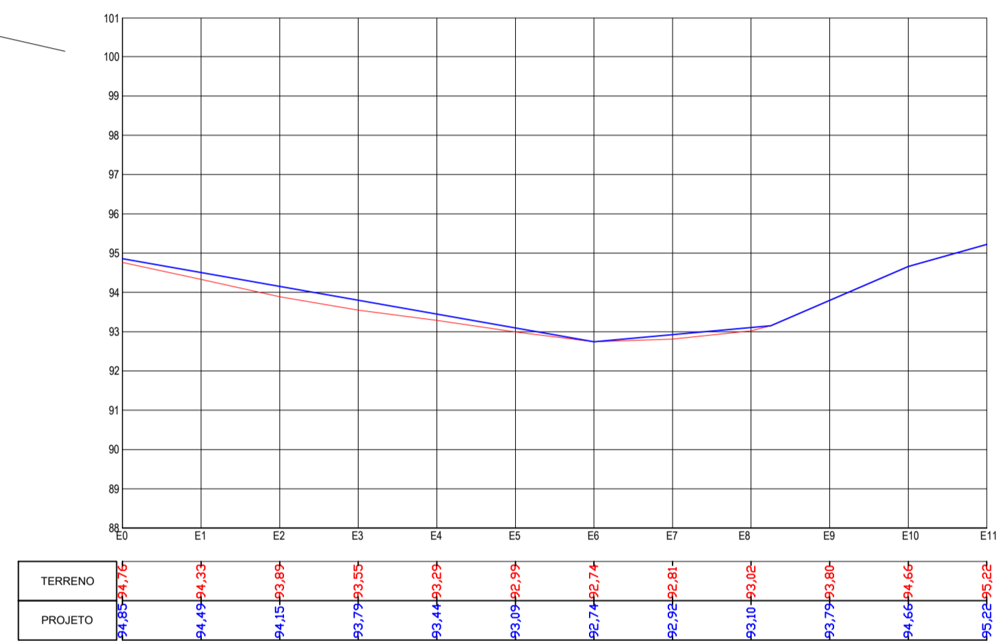
PERFIL RUA 1
