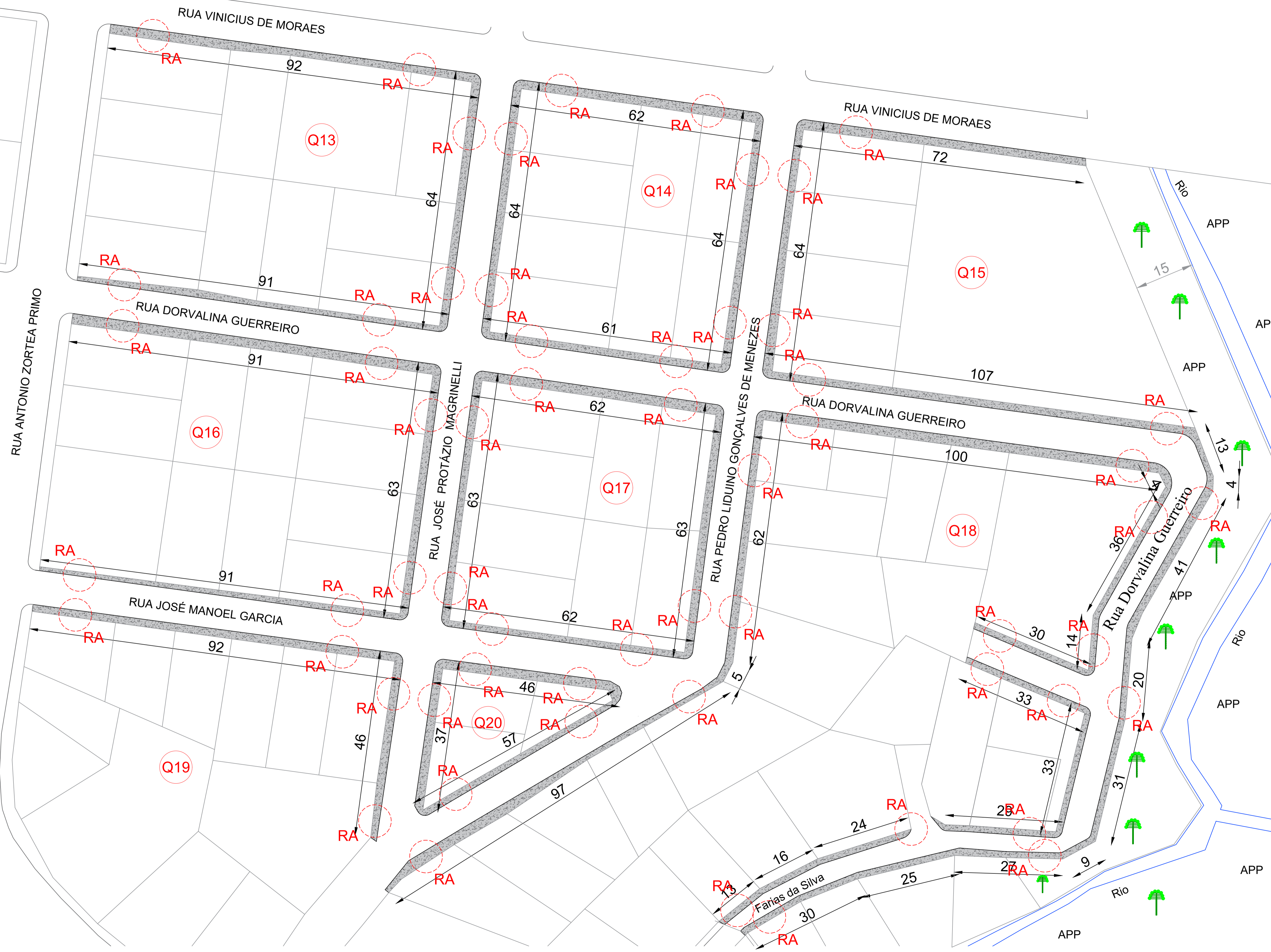
PLANTA BAIXA TÉCNICA DE PASSEIO COM ACESSIBILIDADE TRECHO 03 ESC.: 1:500
