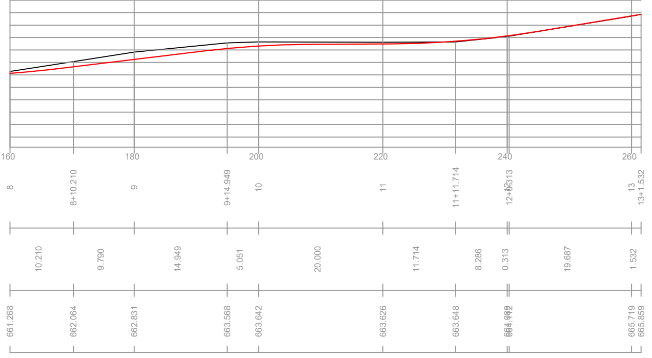
Perfil Longitudinal da Rua Leopoldina
