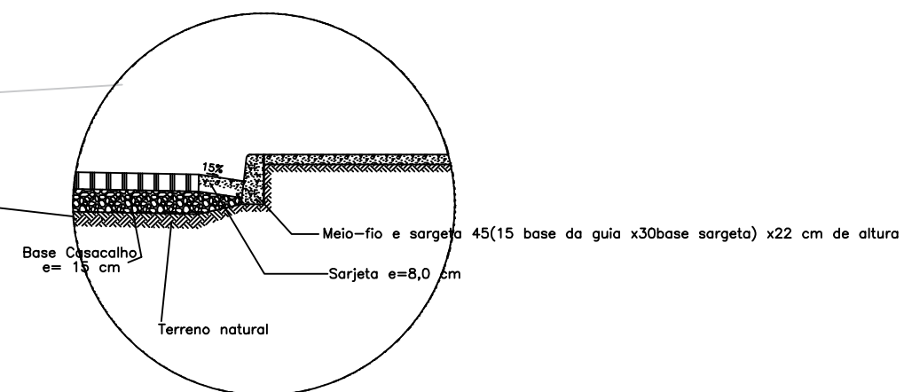
DETALHAMENTO SARJETA SEM ESC.
