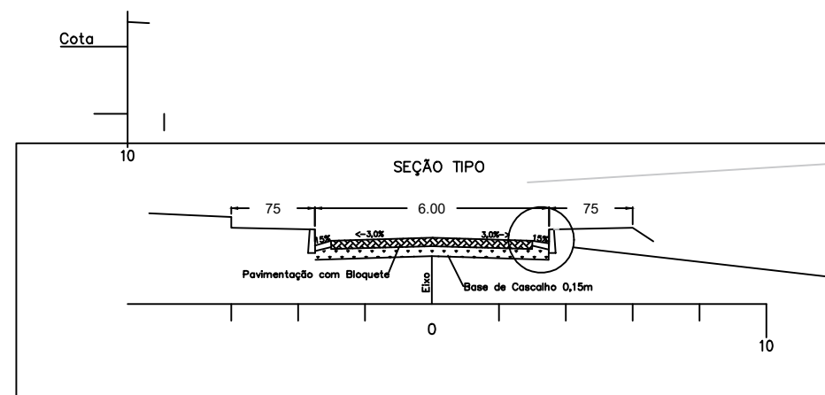
SEÇÃO TRANSVERSAL AVENIDA PRINCIPAL SEM ESCALA
