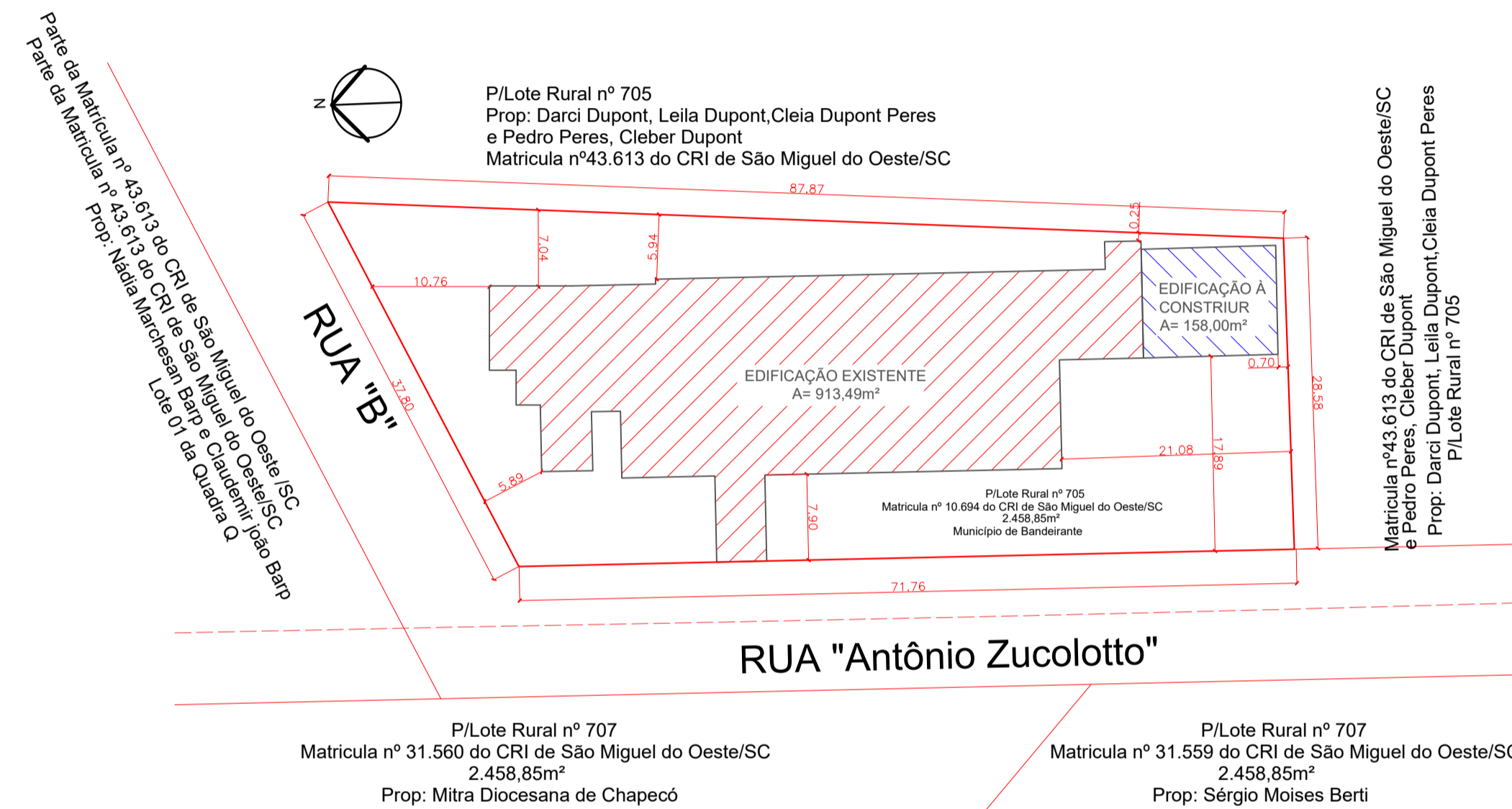
PLANTA DE SITUAÇÃO/LOCAÇÃO ESCALA: 1/500
