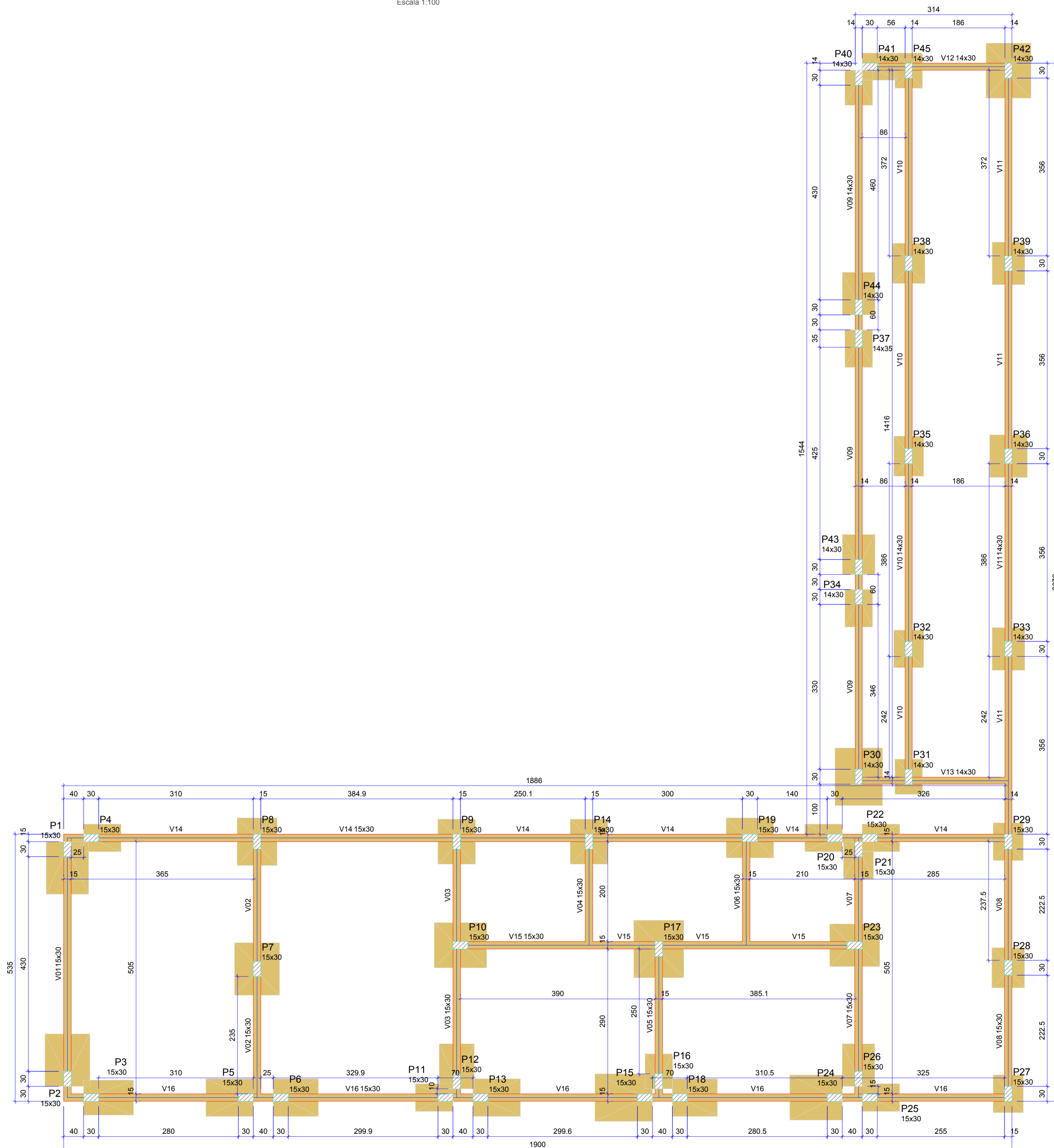
FORMA DO PAVIMENTO BALDRAMES (NÍVEL 0)
