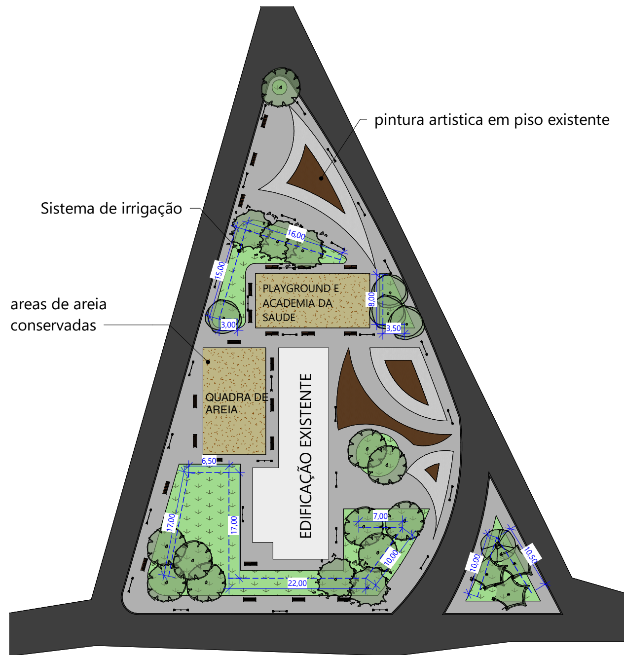
1 PLANTA BAIXA TÉRREO ESCALA 1 : 600
