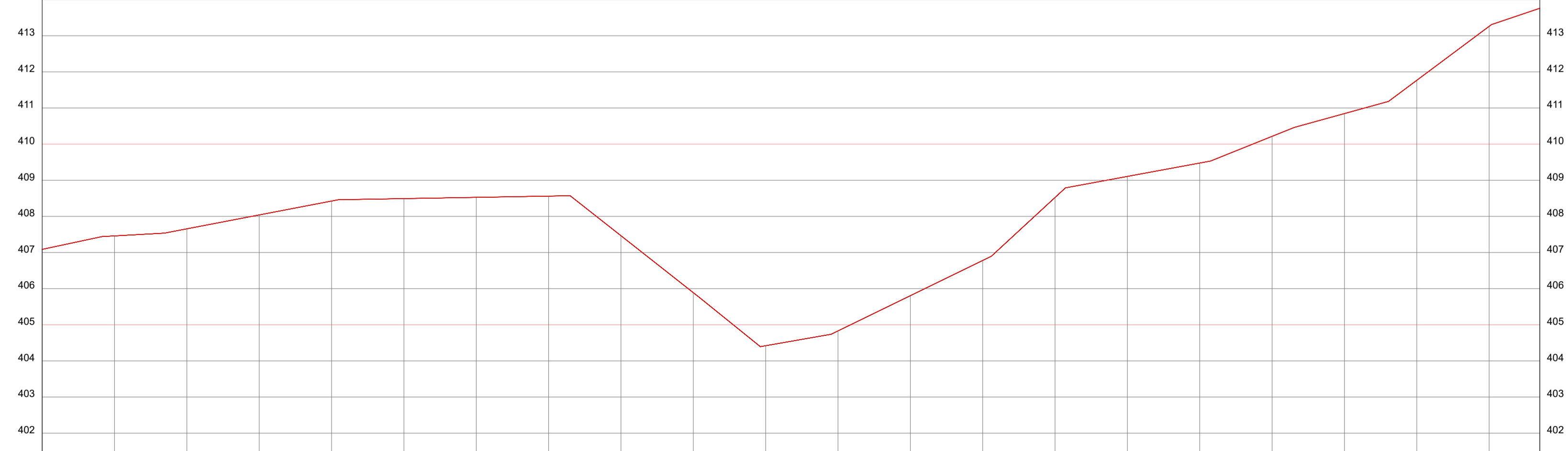
PERFIL LONGITUDINAL RUA JOSÉ FLORENCIO TRECHO 2 Escala Vertical: 1/100 Escala Horizontal: 1/1000
