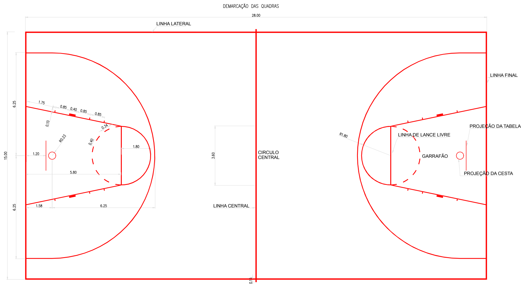
PLANTA DE DETALHAMENTO DA QUADRA DE BASKETEBOL
