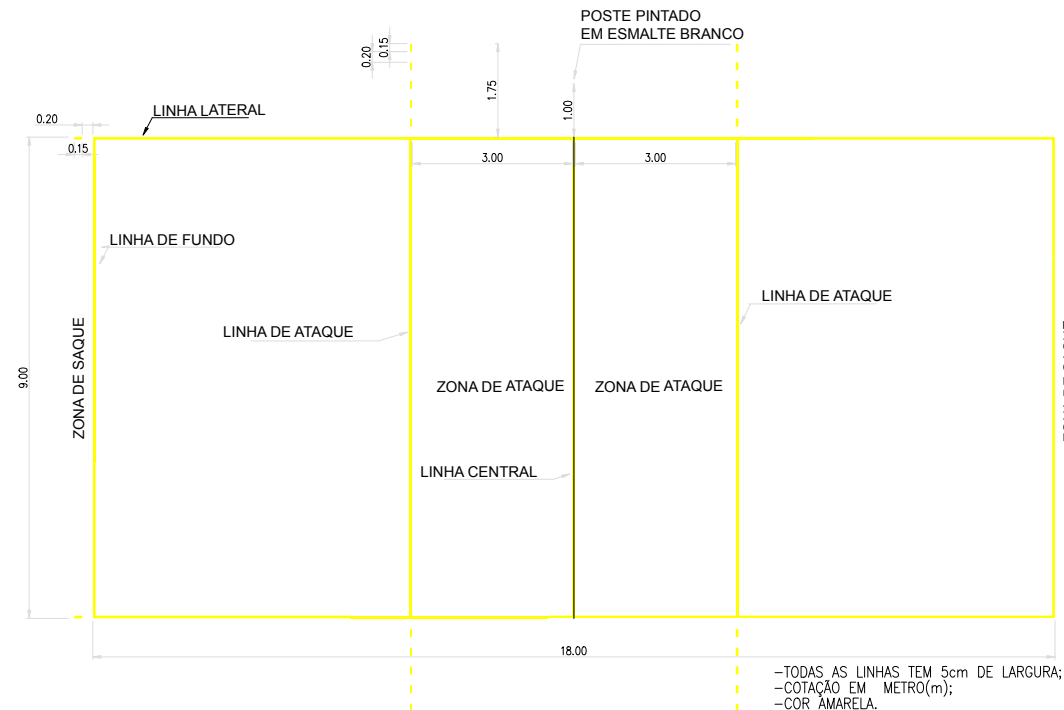
PLANTA DE DETALHAMENTO DA QUADRA DE VOLEIBOL
