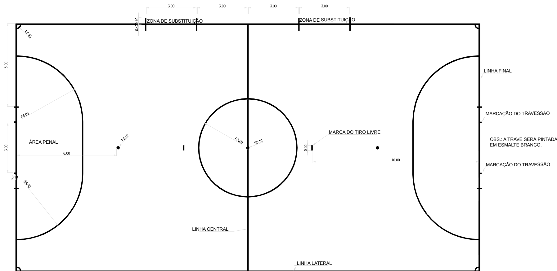
PLANTA DE DETALHAMENTO DA QUADRA DE FUTSAL
