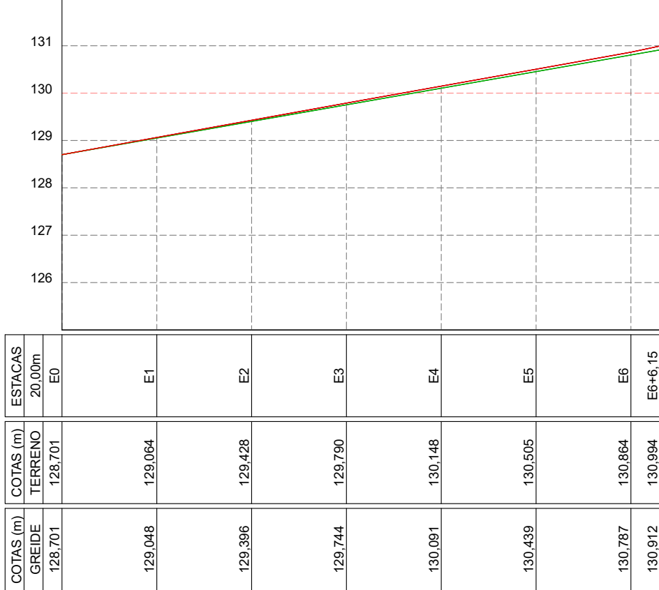
PERFIL LONGITUDINAL TRECHO 2 - LOC. PINTADO ESCALA VERTICAL: 1/100 ESCALA HORIZONTAL: 1/1000
