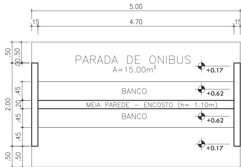
PLANTA CONSTRUTIVA esc 1:50
