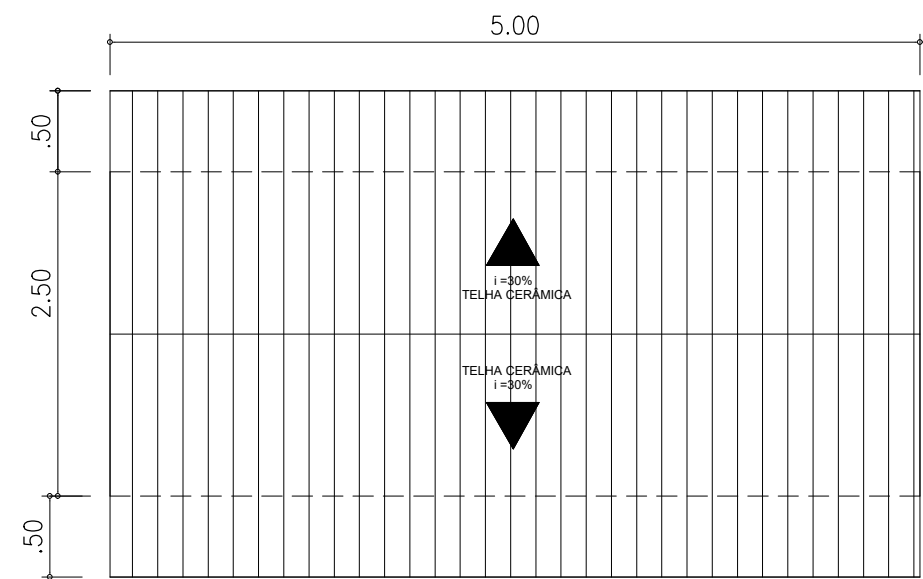
PLANTA DE COBERTURA esc 1:50
