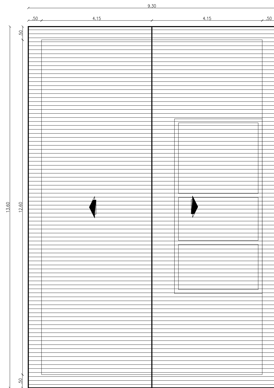
PLANTA BAIXA COBERTURA esc 1:75
