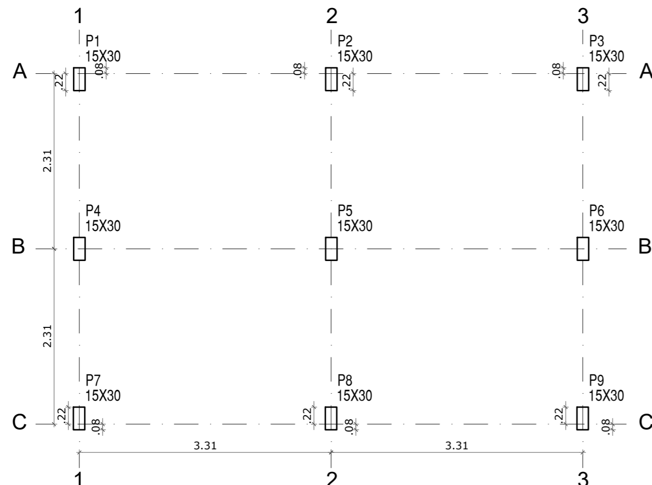
PLANTA DE LOCAÇÃO DOS PILARES BANHEIROS ESC 1/50
