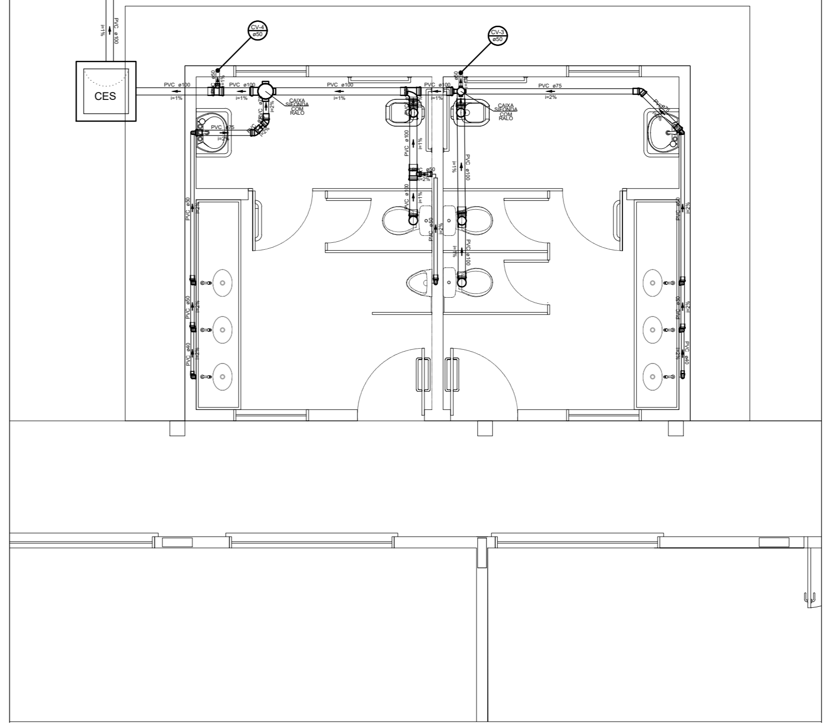
PLANTA BAIXA SANITÁRIA BANHEIROS SOCIAIS ESC 1/50
