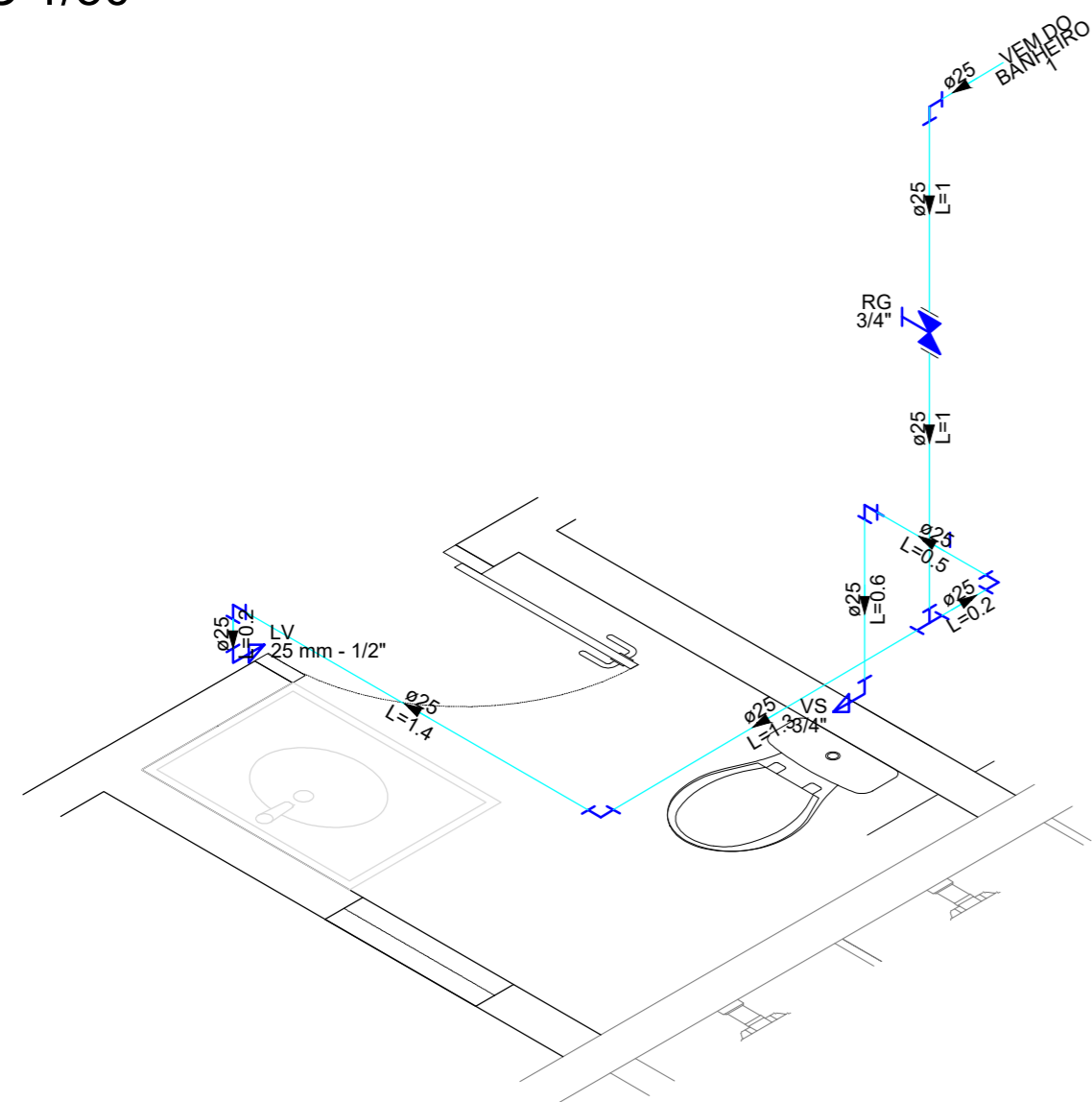
◁ DETALHE H2 1:25
