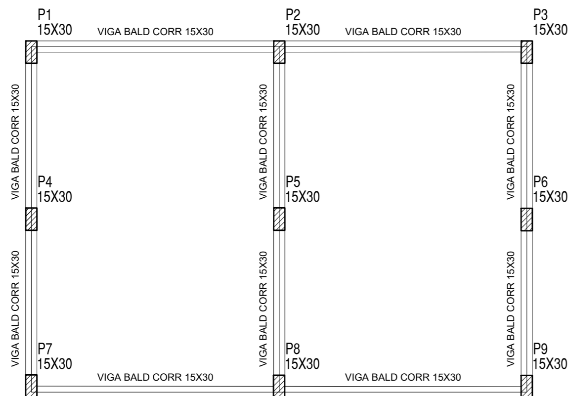
PLANTA DE FORMA PAV. TERREO BANHEIROS ESC 1/50
