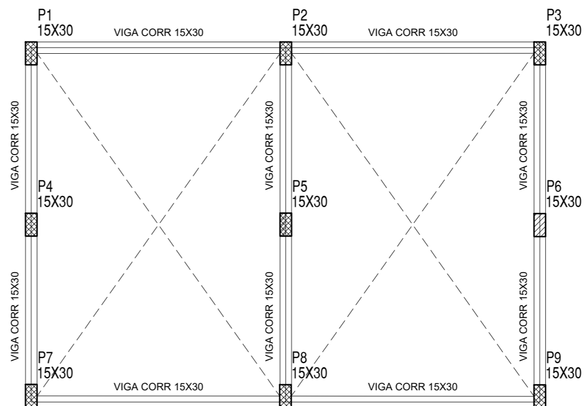
PLANTA DE FORMA NIVEL +330 BANHEIROS ESC 1/50
