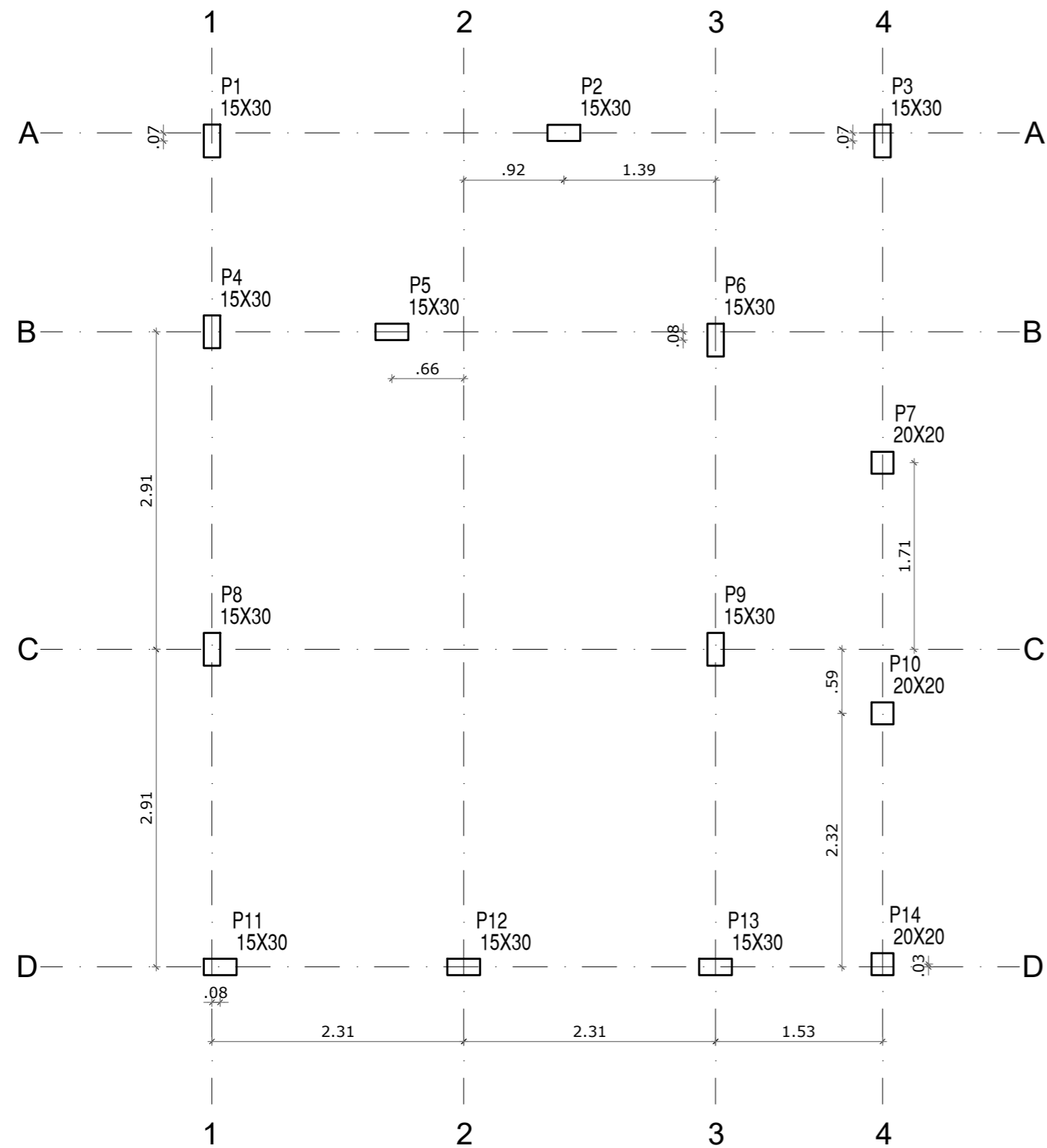
PLANTA DE LOCAÇÃO DOS PILARES SALA DOS PROFESSORES ESC 1/50
