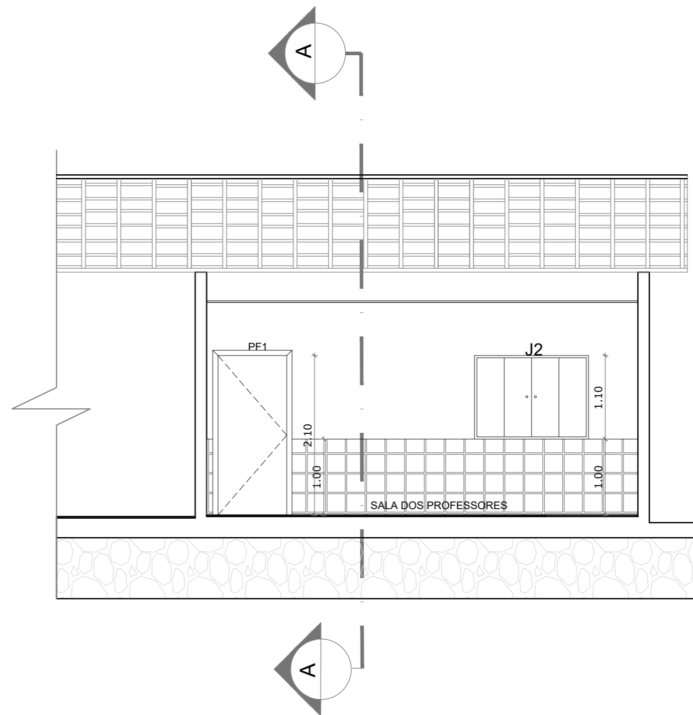
CORTE BB AMPLIAÇÃO SALA DOS PROFESSORES ESC 1/50
