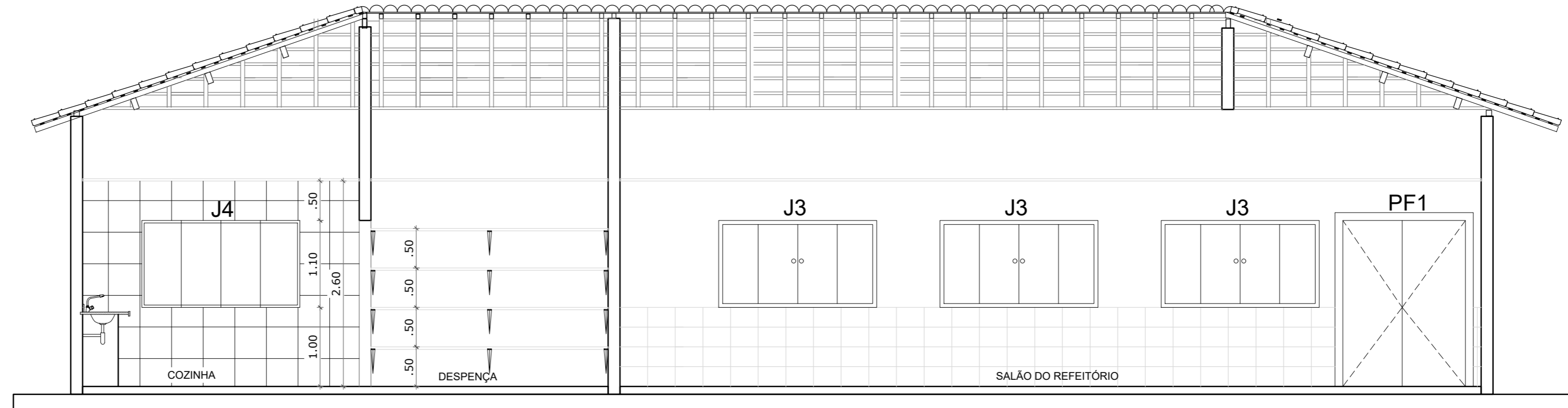
CORTE CC AMPLIAÇÃO REFEITÓRIO ESC 1/50
