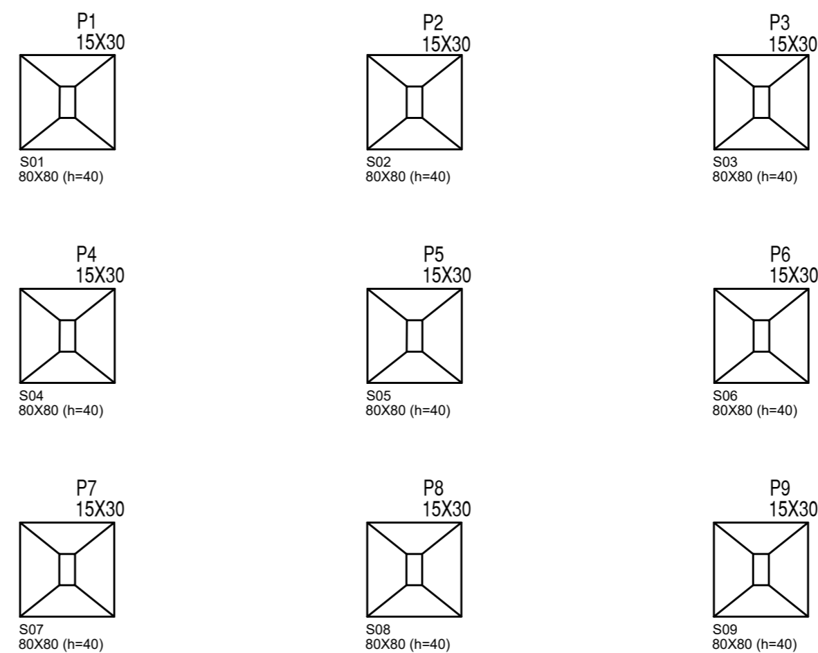
PLANTA DE LOCAÇÃO DAS FUNDAÇÕES SBANHEIROS ESC 1/50
