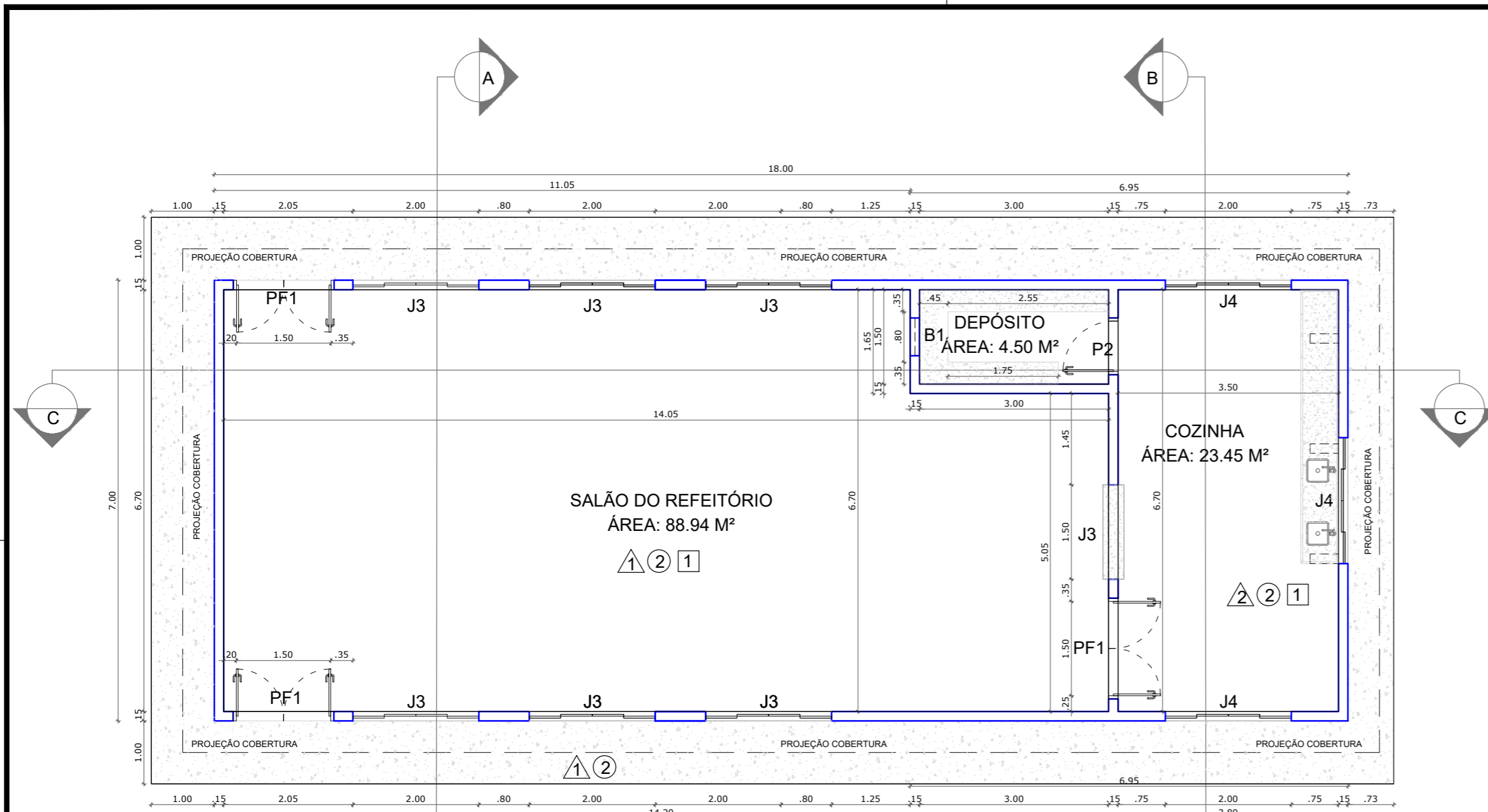
PLANTA BAIXA AMPLIAÇÃO REFEITÓRIO ESC 1/75
