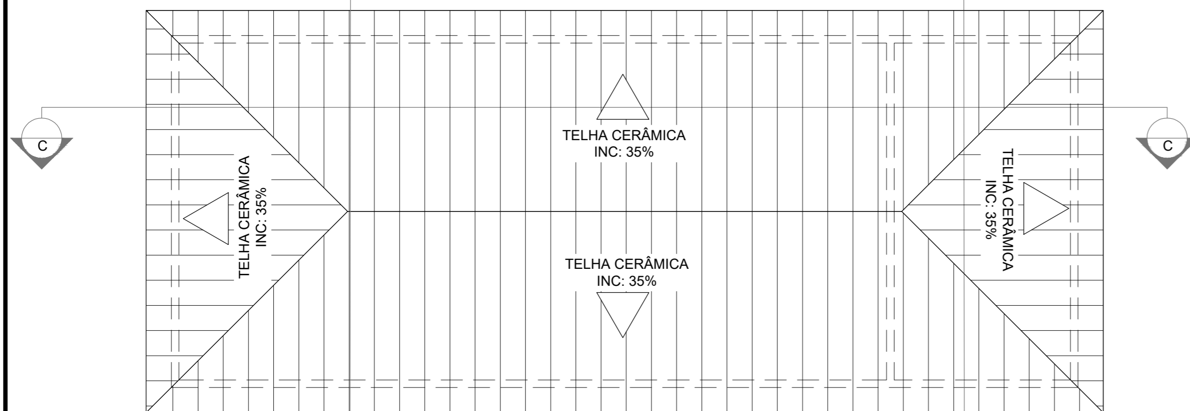
PLANTA COBERTURA AMPLIAÇÃO REFEITÓRIO ESC 1/75
