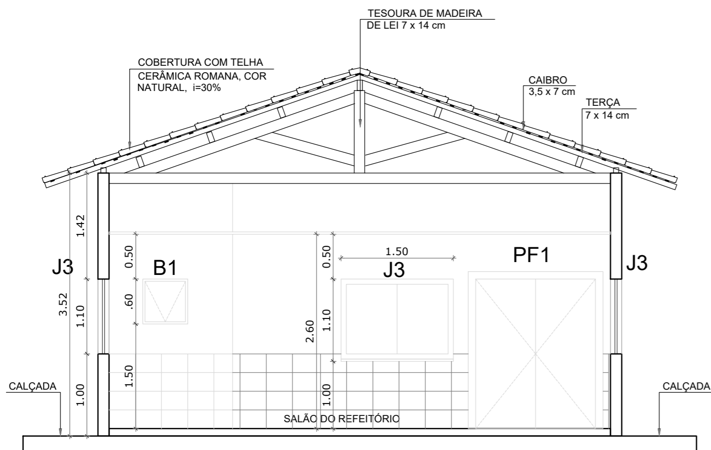
CORTE AA AMPLIAÇÃO REFEITÓRIO ESC 1/50
