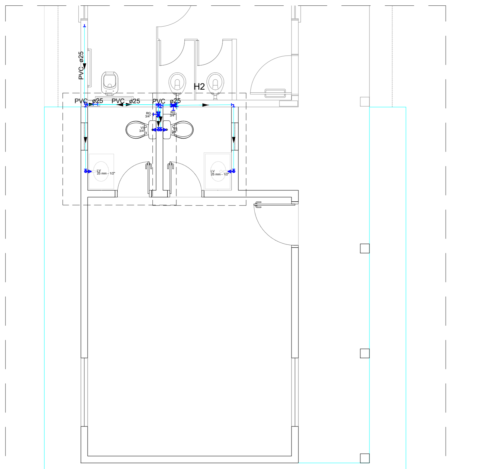
PLANTA BAIXA HIDRAULICA ESC 1/50
