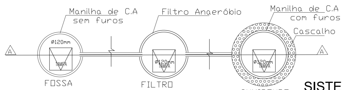
ESQUEMA DE TRATAMENTO DE ESGOTO
