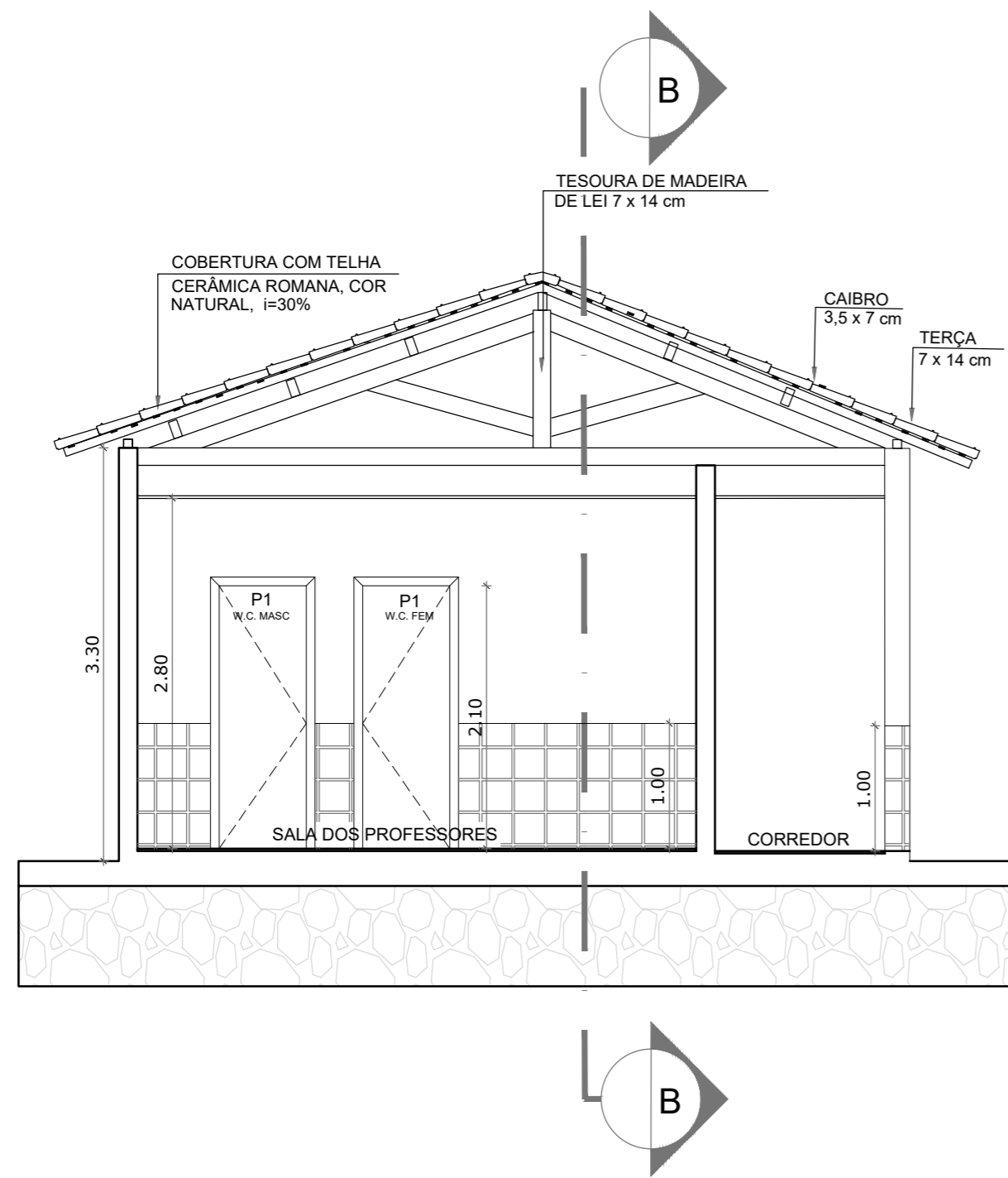
CORTE AA AMPLIAÇÃO SALA DOS PROFESSORES ESC 1/50
