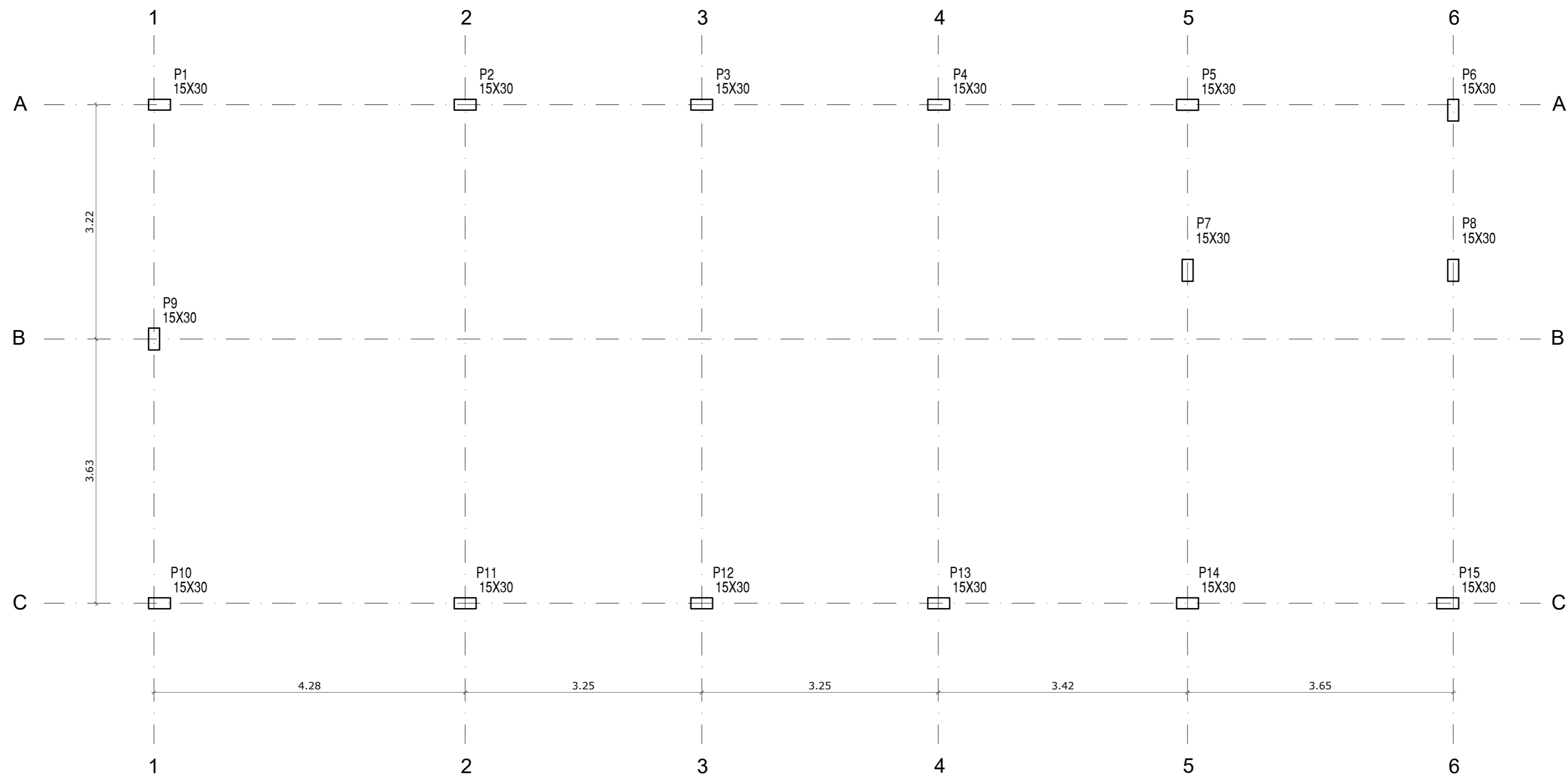
PLANTA DE LOCAÇÃO DOS PILARES REFEITORIO ESC 1/50
