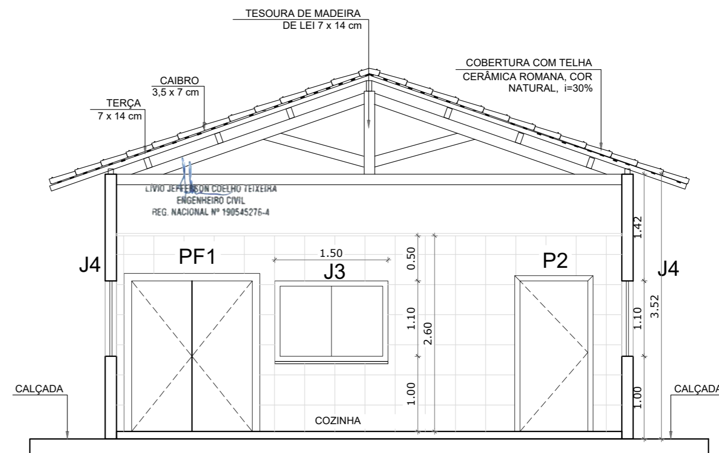
CORTE BB AMPLIAÇÃO REFEITÓRIO ESC 1/50
