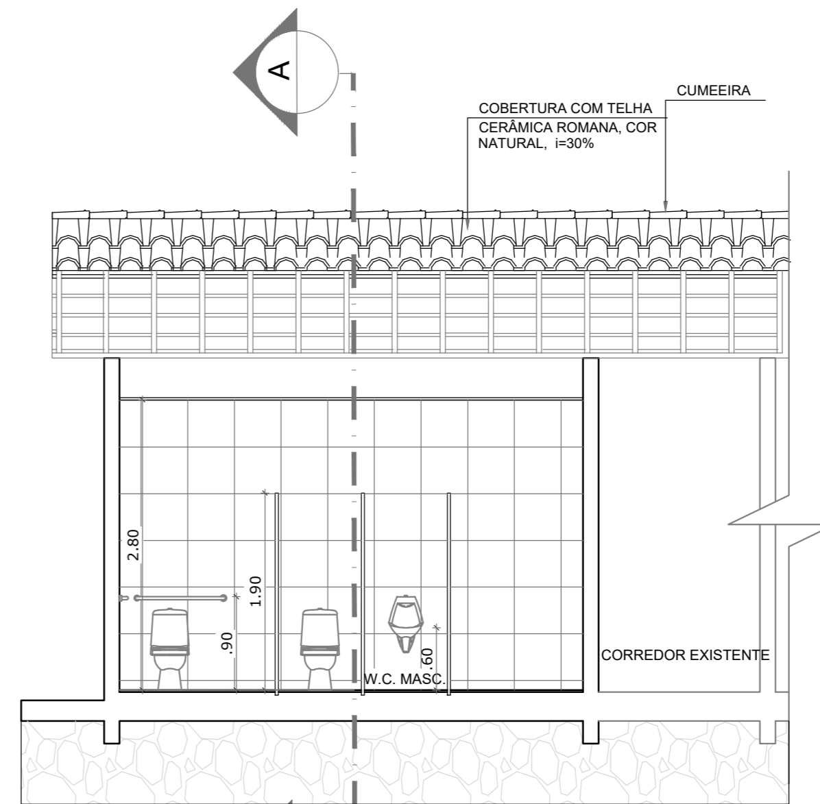
CORTE BB AMPLIAÇÃO BANHEIROS ESC 1/50
