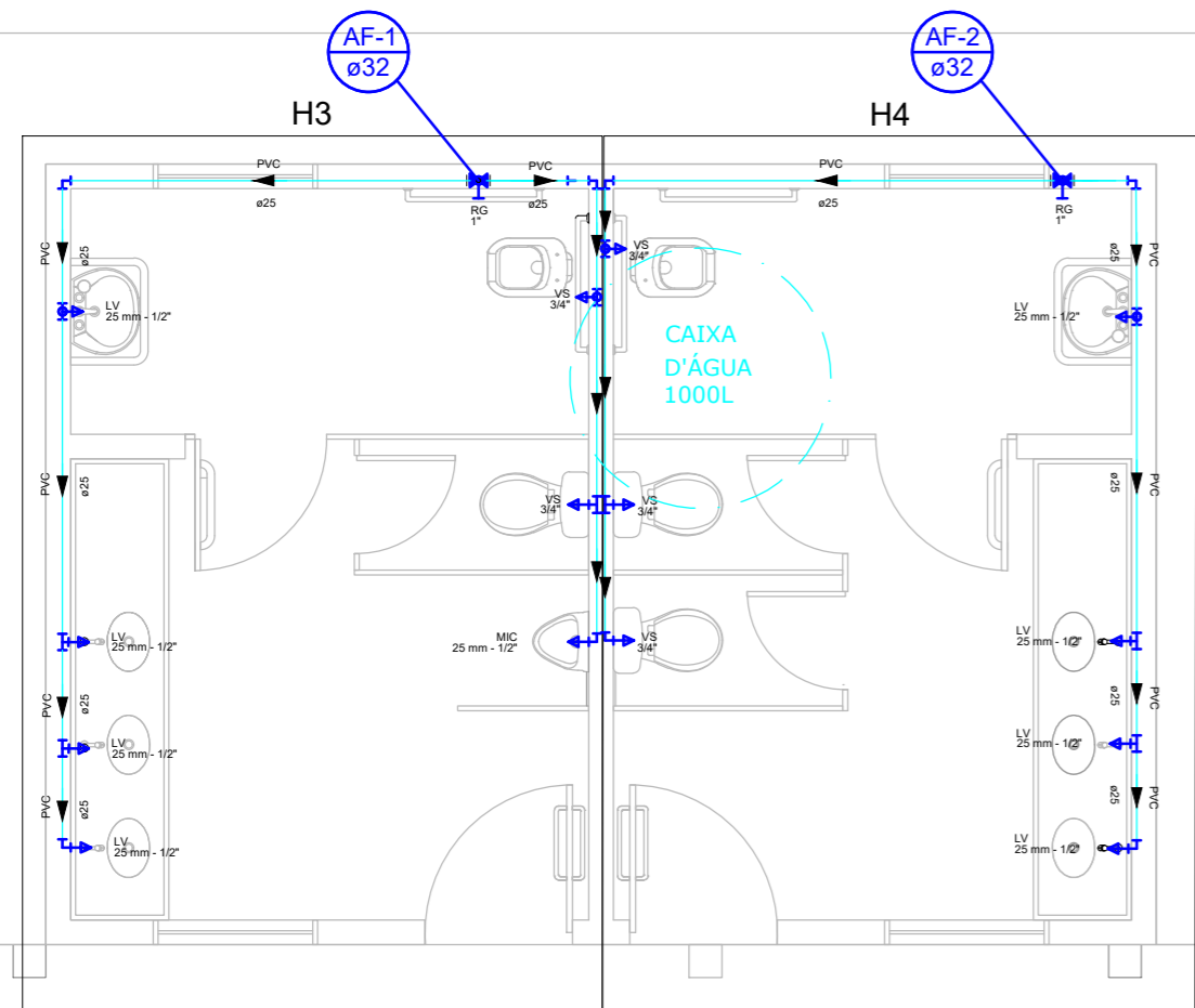
PLANTA BAIXA HIDRAULICA ESC 1/50
