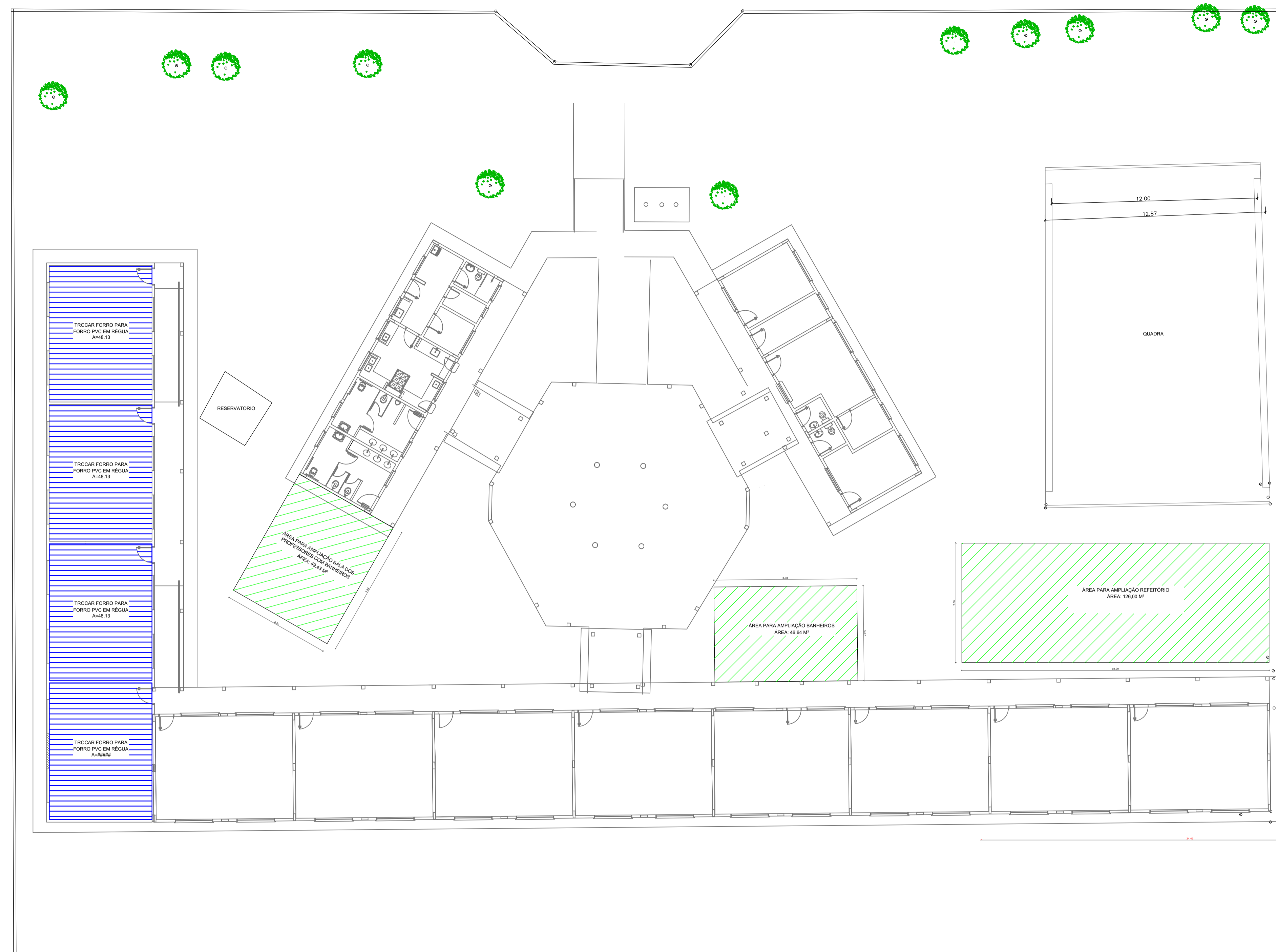
PLANTA BAIXA EXISTENTE ESCALA 1/150
