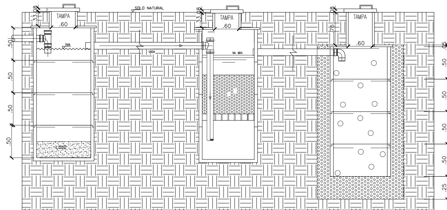
CORTE A-A
