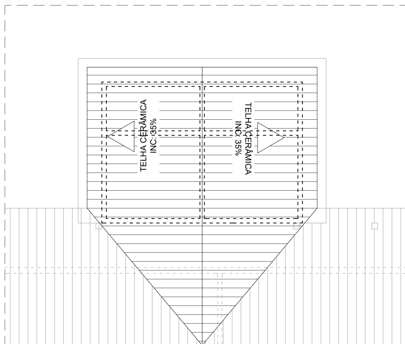
PLANTA COBERTURA AMPLIAÇÃO SALA DOS BANHEIROS ESC 1/75
