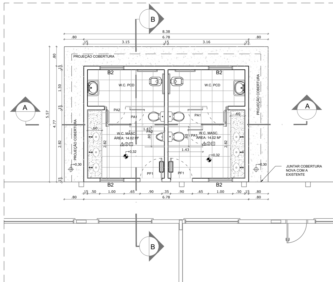
PLANTA BAIXA AMPLIAÇÃO SALA DOS BANHEIROS ESC 1/75
