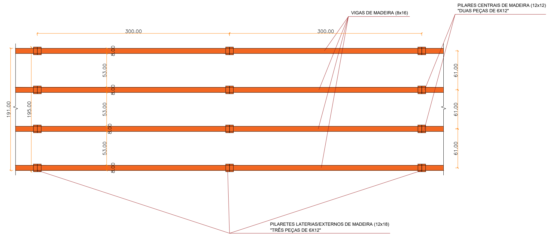
DETALHE VIGAS E PILARES DO DECK - VISTA SUPERIOR
