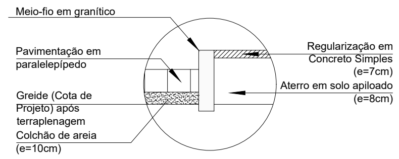
Detalhe 01 Escala — 1:25
