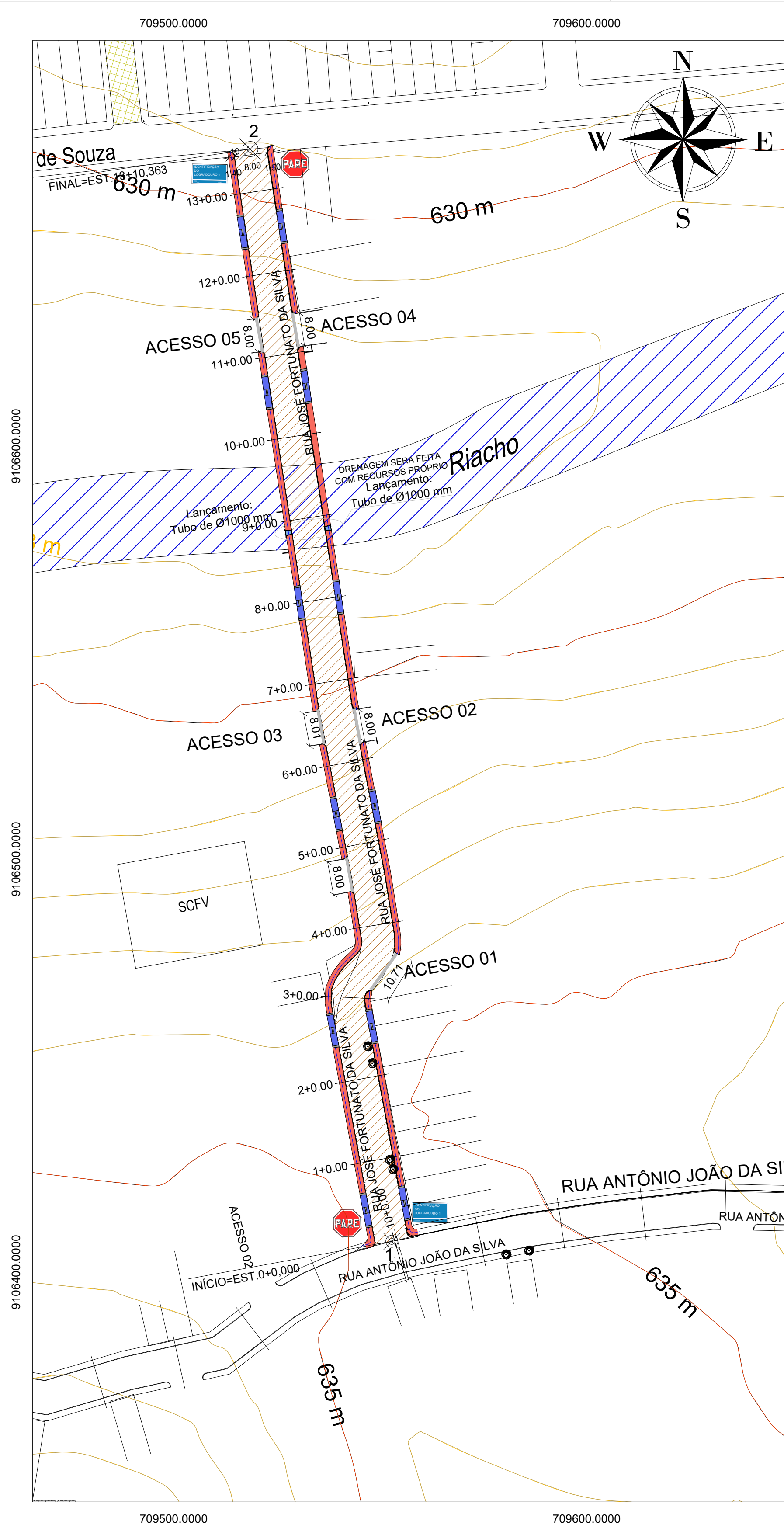
Planimetria Escala — 1/800
