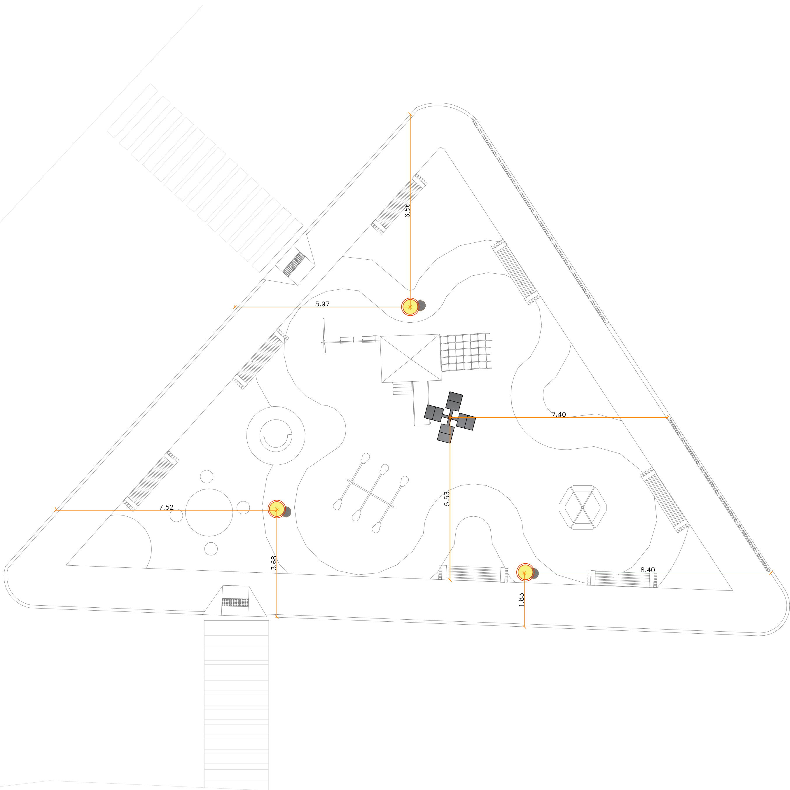
PLANTA DE ILUMINAÇÃO - LOCAÇÃO DE POSTES Esc.: 1/75
