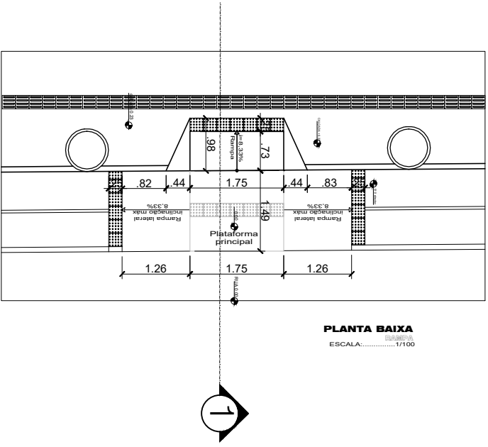
RAMPA DE ACESSIBILIDADE
