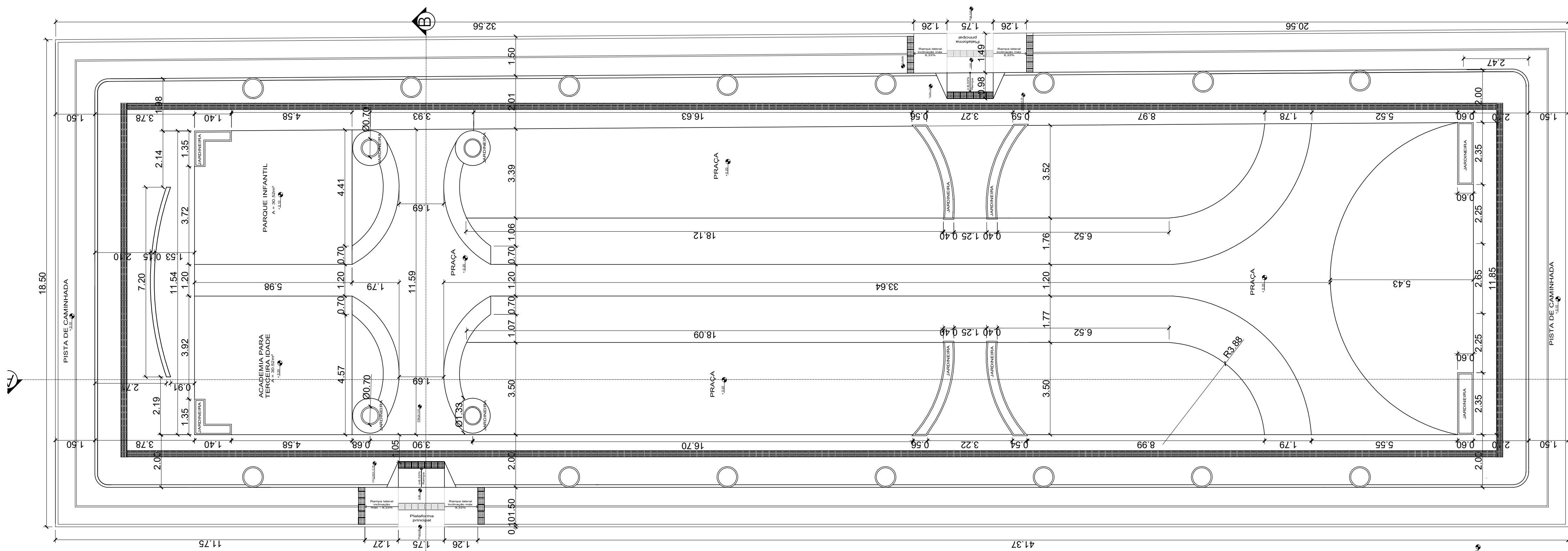
PLANTA BAIXA- PRAÇA ESCALA:.....1/100
