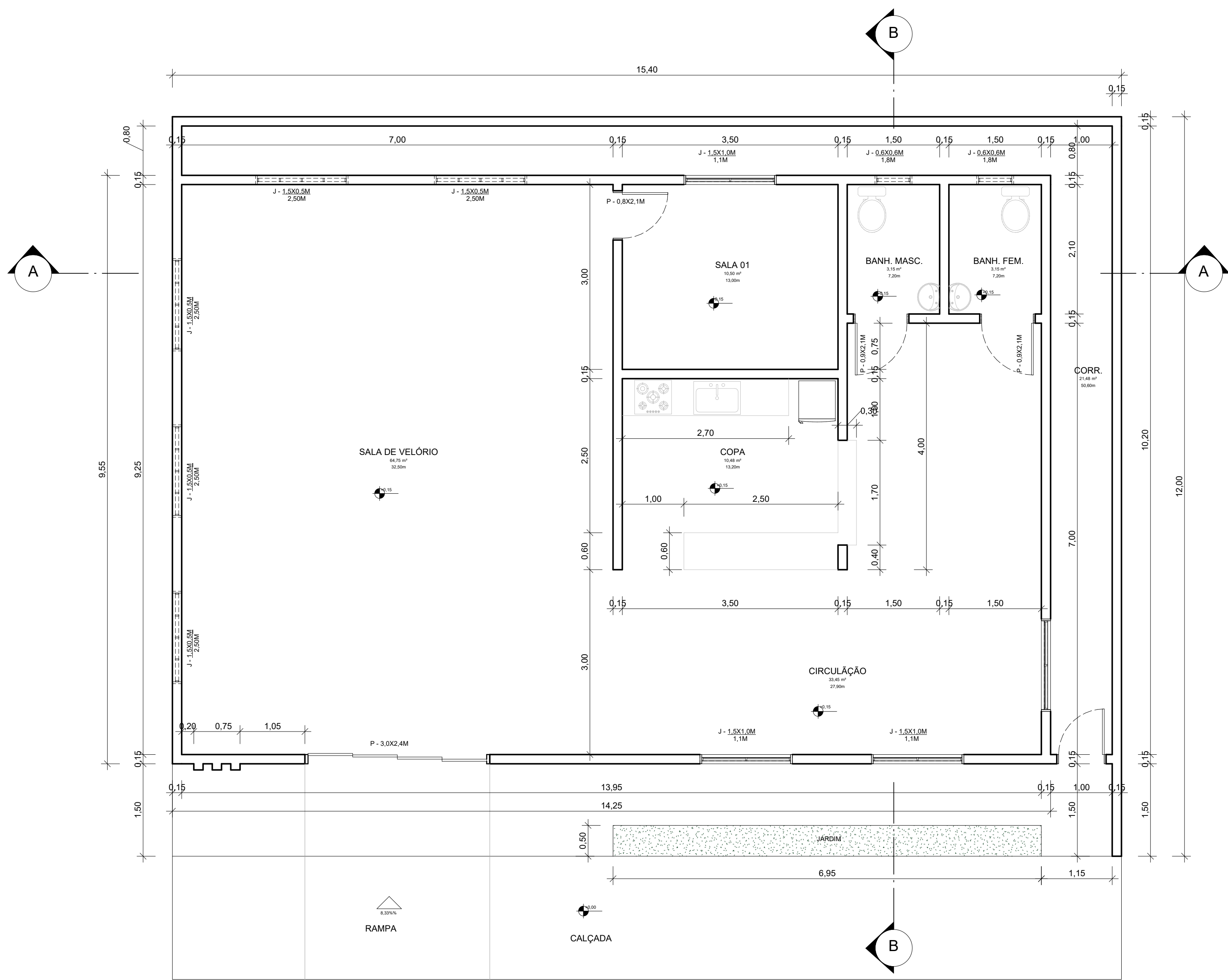
1 PLANTA BAIXA SALA DE VELÓRIO Escala: 1 : 50
