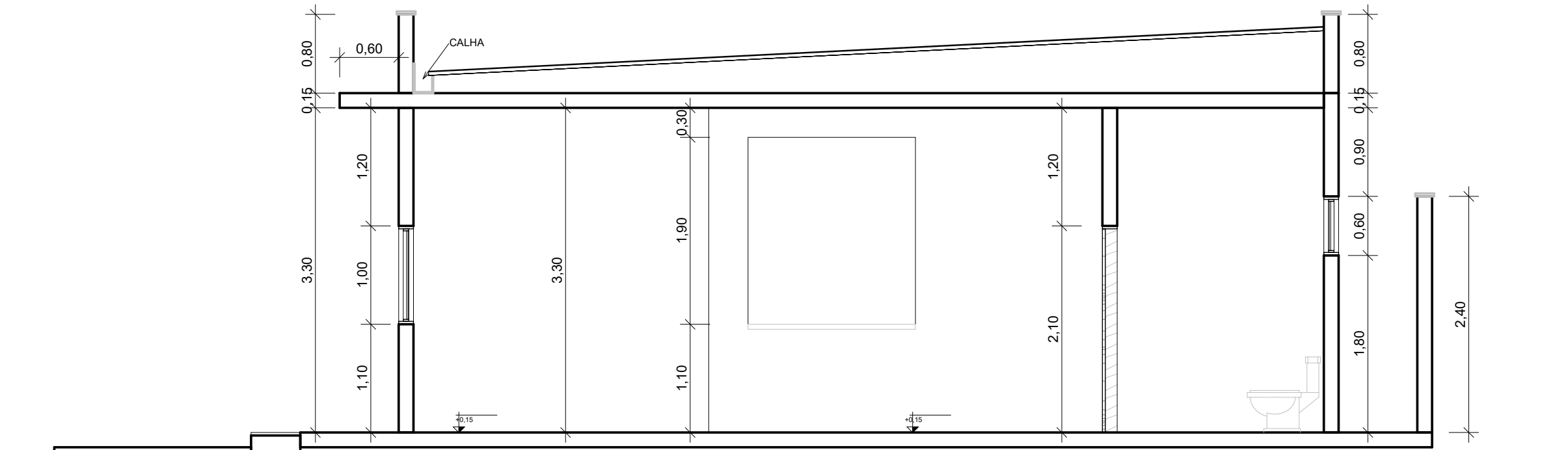
3 CORTE BB Escala: 1 : 50
