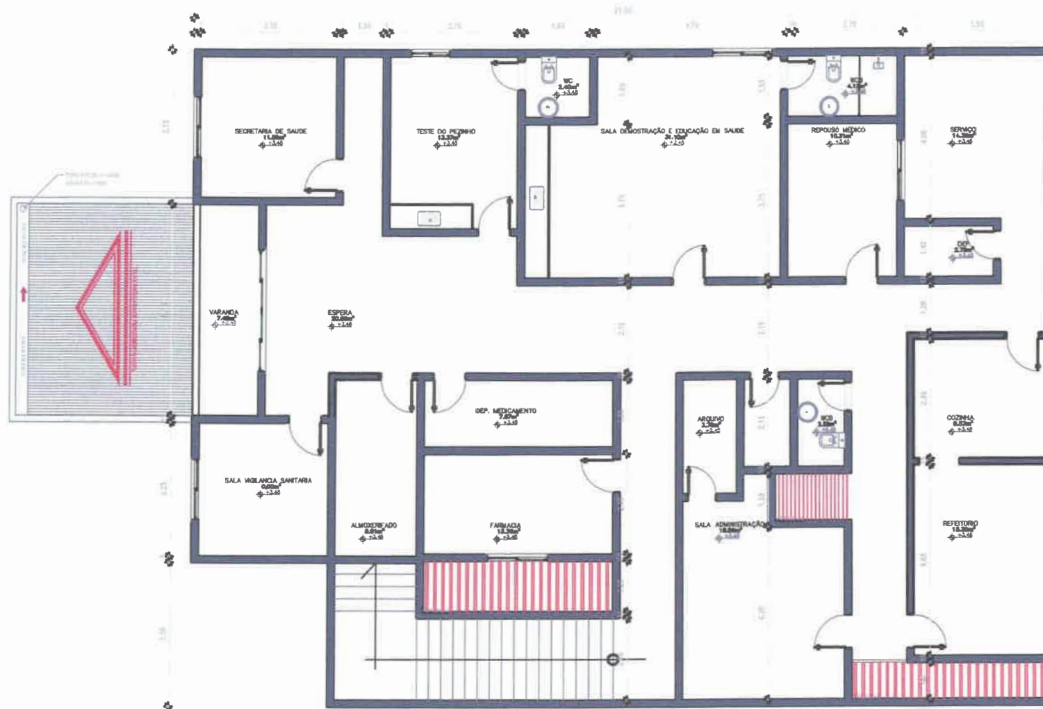
PLANTA 1ª PAV SITUAÇÃO ATUAL — POLICLINICA ESC. 1/75
