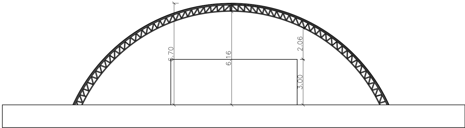
VISTA FRONTAL - COBERTURA PRAÇA Escala 1:25
