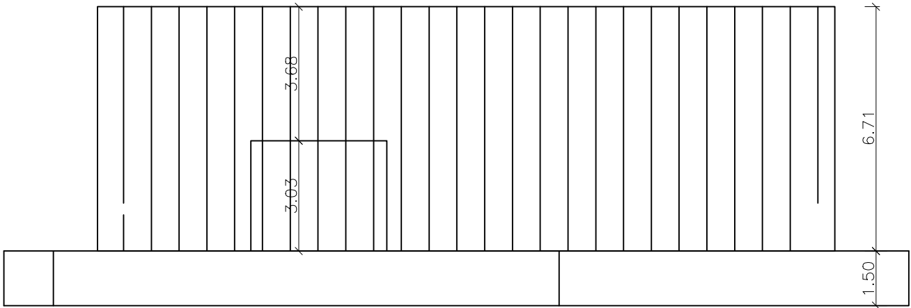
VISTA LATERAL - COBERTURA PRAÇA Escala 1:25
