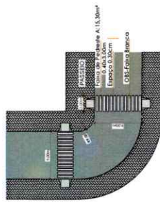
DETALHE INTERSEÇÃO - FAIXA DE PEDESTRE ESCALA 1:300 ÁREA DE PINTURA FAIXA DE PEDESTRE INDIVIDUAL: 15,60m²
