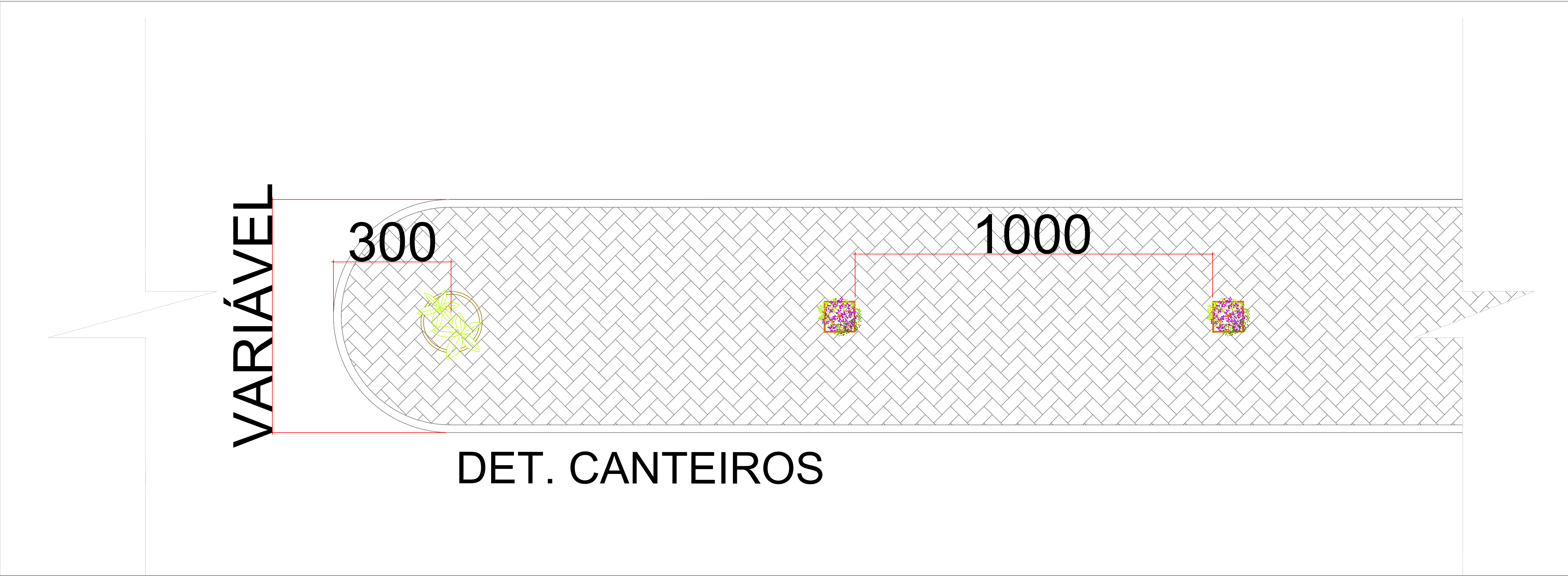
AV. VITÓRIO SEGUNDO BEN ESC: 1:75
