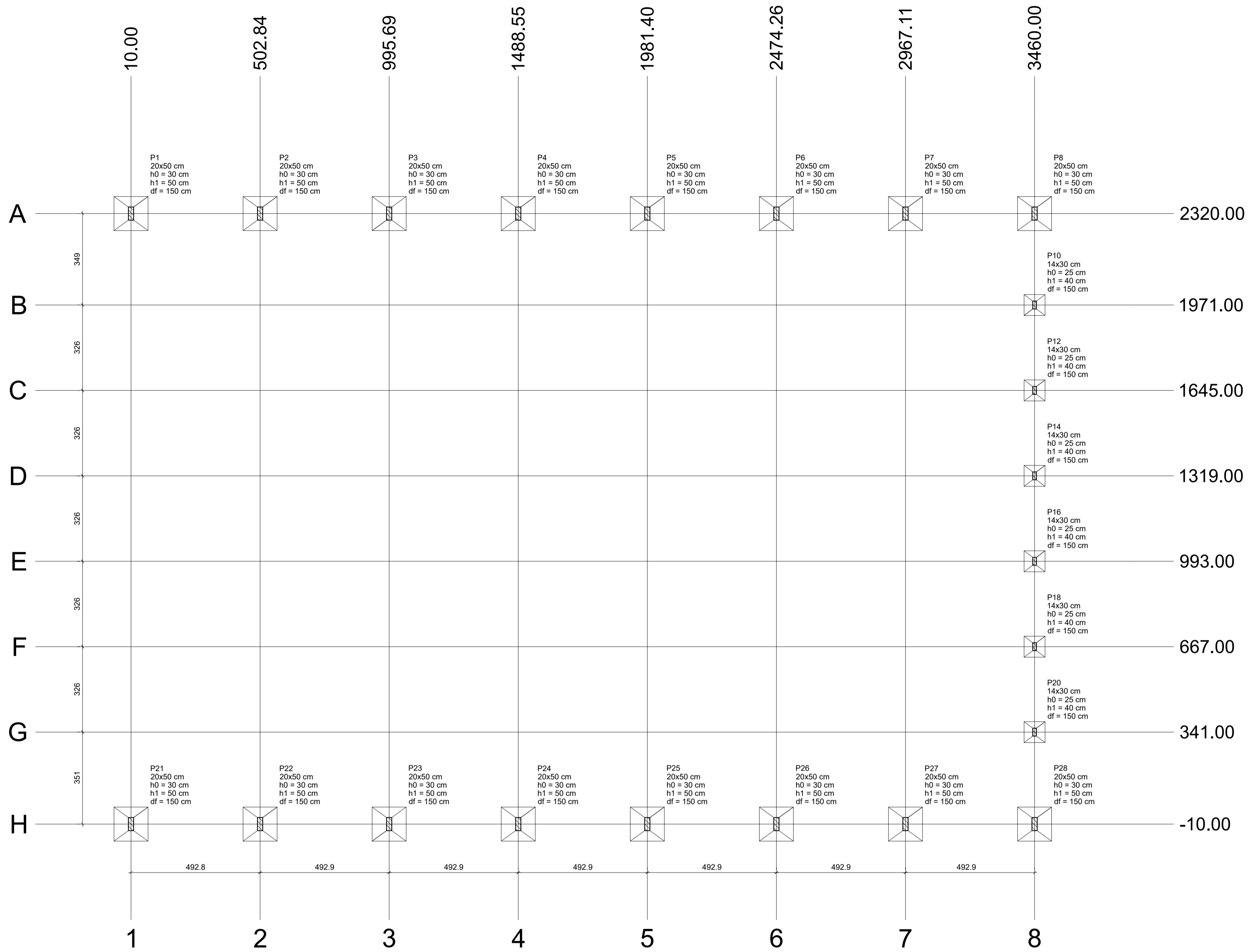
Planta de locação escala 1:100
