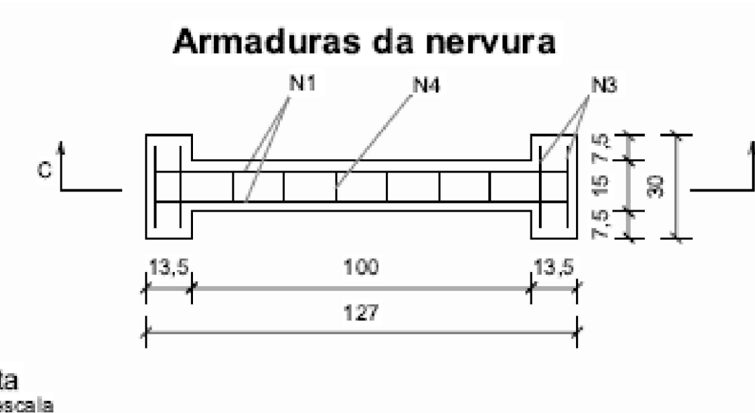
Corte C-C' Sem escala
