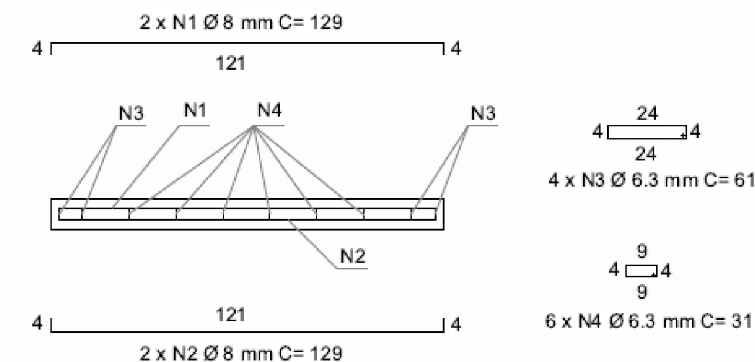
Corte C-C' Sem escala
