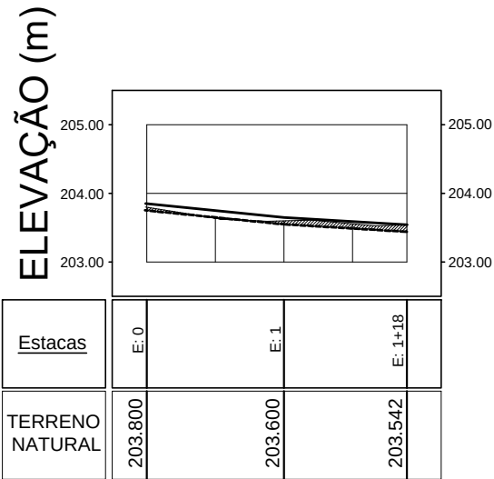
PERFIL - Rua Alcina Maria, T-1 Escala Vertical: 100 Horizontal:1000
