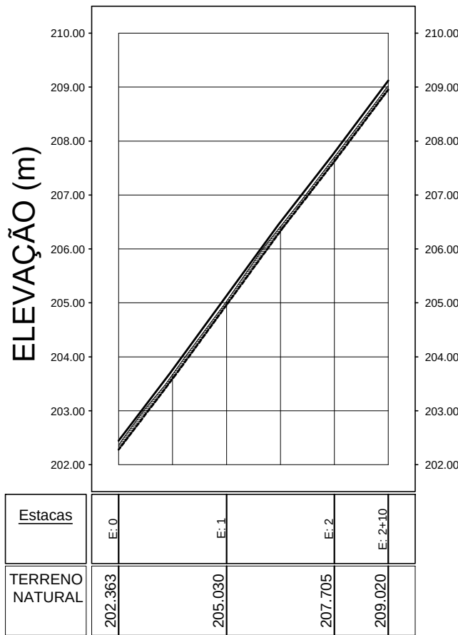
PERFIL - Rua Cirilo José de Lima Escala Vertical: 100 Horizontal:1000
