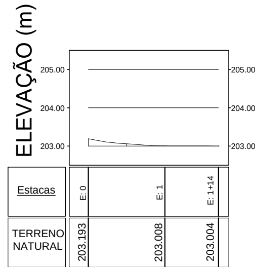
PERFIL - Rua Antonio Serafim de Lima Escala Vertical: 100 Horizontal:1000
