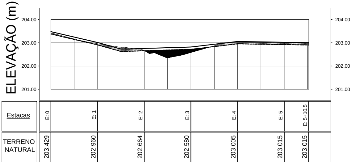
PERFIL - Rua Alcina Maria, T-2 Escala Vertical: 100 Horizontal:1000
