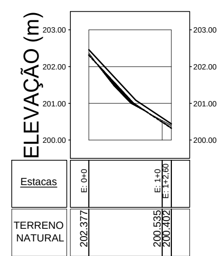
PERFIL - Rua Antonio Cirilo de Lima Escala Vertical: 100 Horizontal:1000
