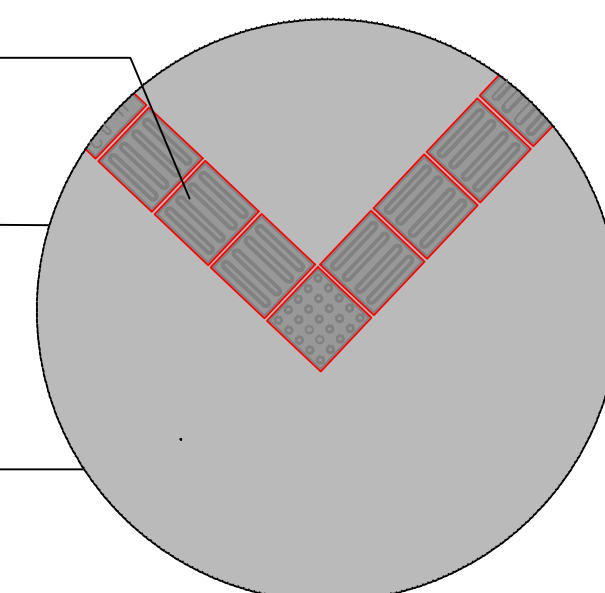
DETALHE: ROTA ACESSÍVEL PAVIMENTAÇÃO ESCALA 1/50
