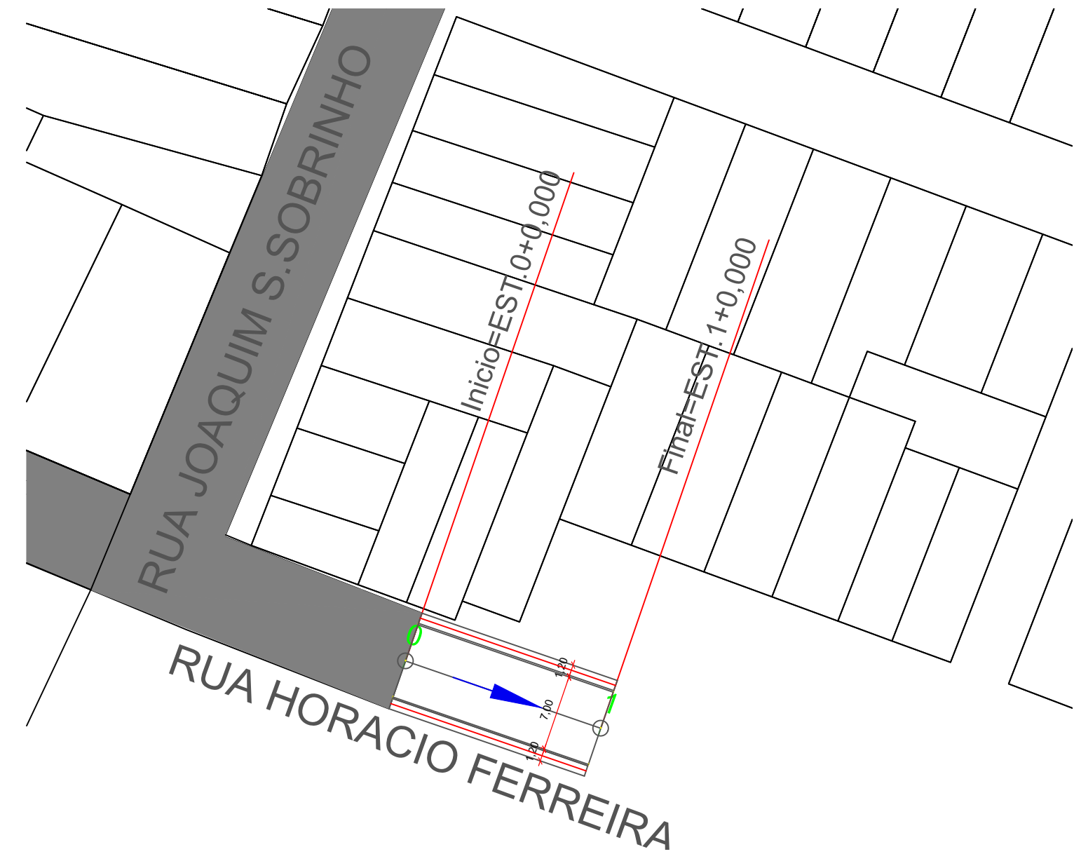
PLANTA BAIXA - RUA HORÁCIO FERREIRA PAVIMENTAÇÃO 1/500
