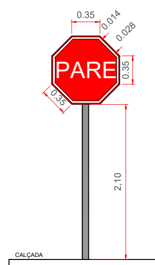
PLACA DE SINALIZAÇÃO - PARADA OBRIGATÓRIA PAVIMENTAÇÃO ESCALA 1/50
