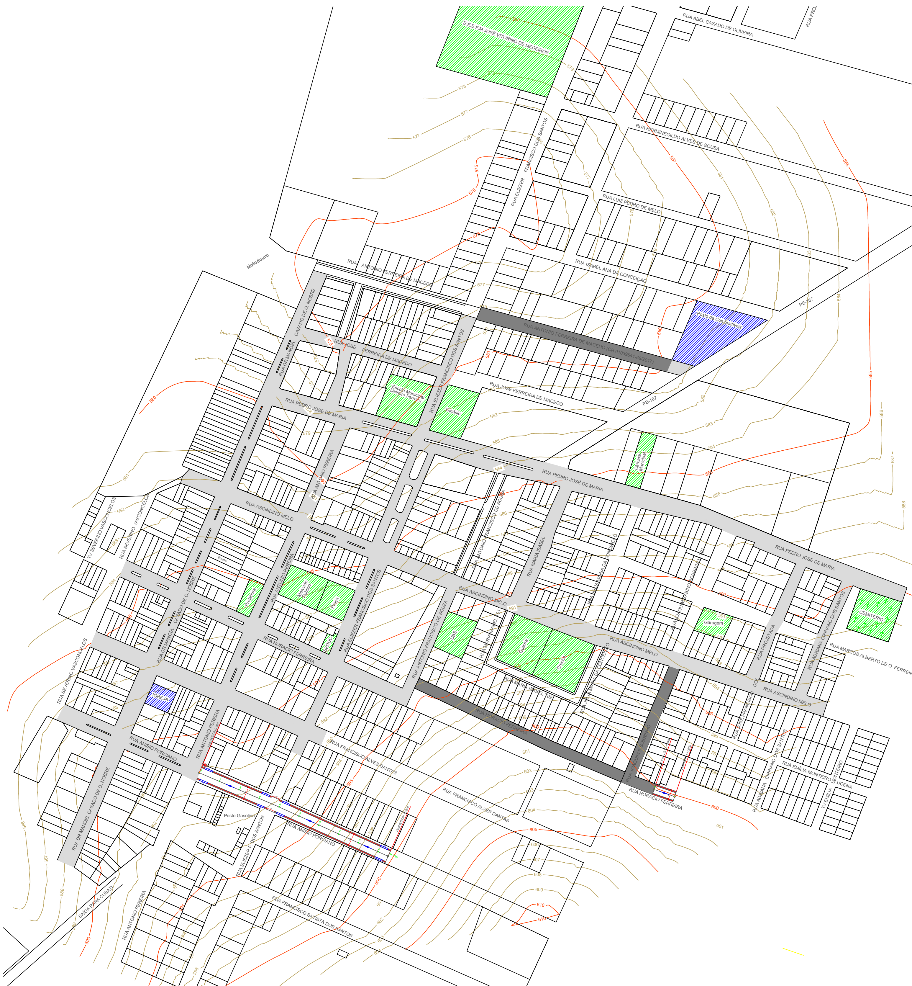
MAPA DE LOCALIZAÇÃO PAVIMENTAÇÃO ESCALA 1/2.000
