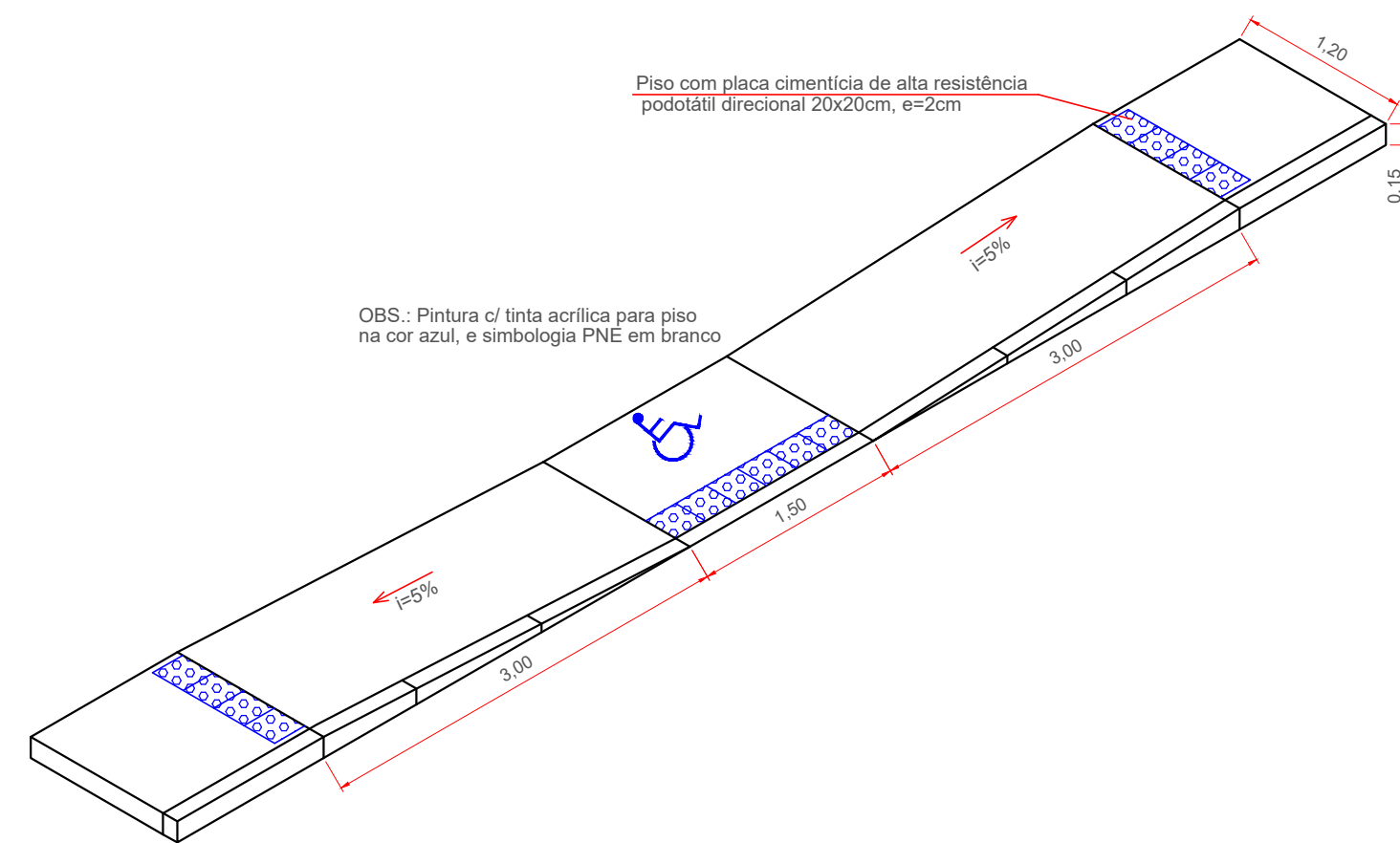
DETALHE: RAMPA DE ACESSIBILIDADE PAVIMENTAÇÃO ESCALA 1/50
