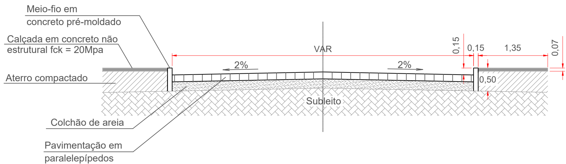
DETALHE: SEÇÃO TRANSVERSAL TIPO PAVIMENTAÇÃO ESCALA 1/50
