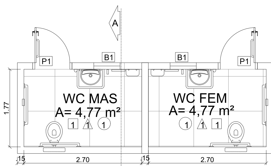
PLANTA BAIXA - WC esc. 1:75
