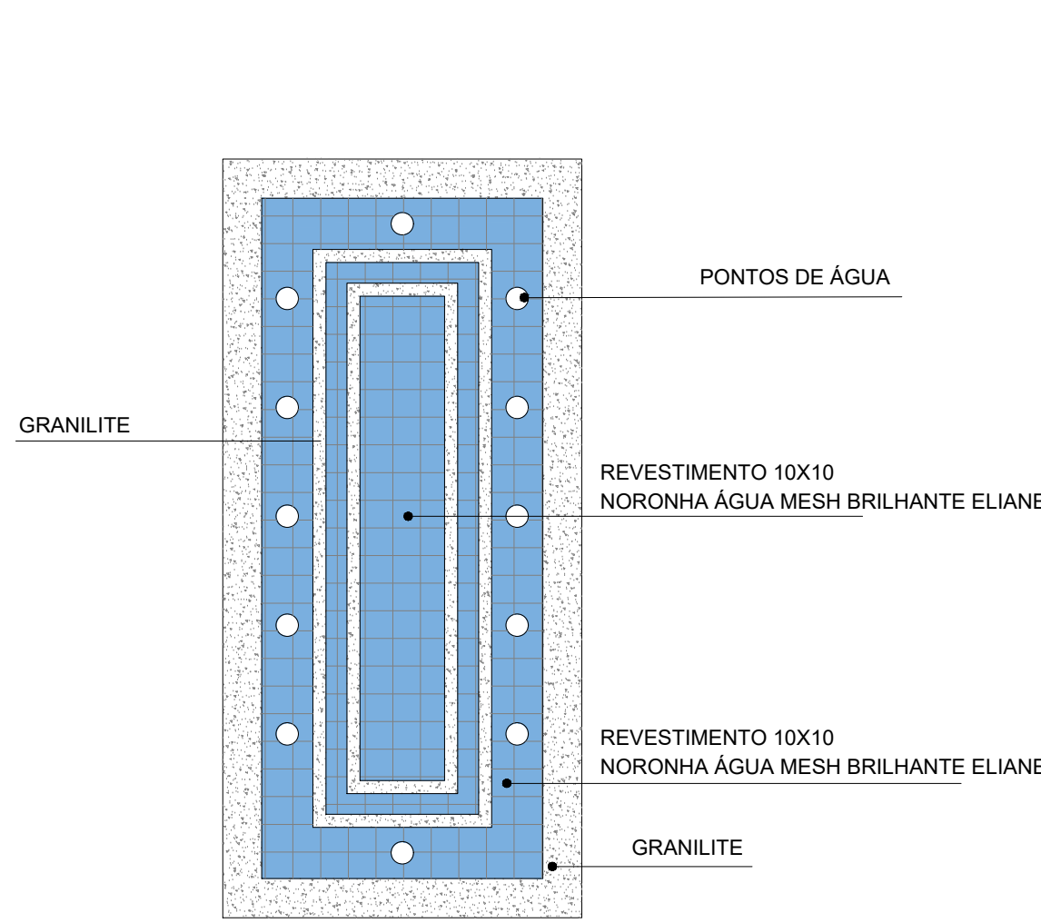
PLANTA PAGINAÇÃO - FONTE esc. 1:75
