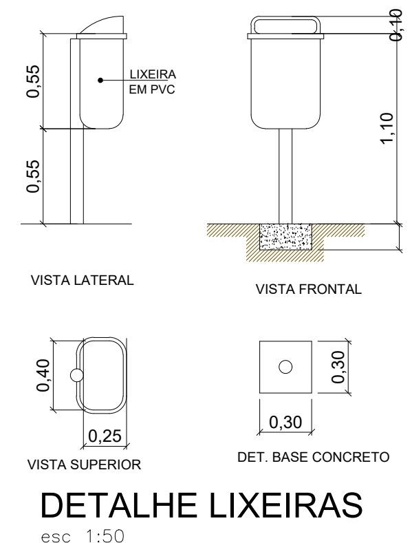
DETALHE LIXEIRAS esc. 1:50
