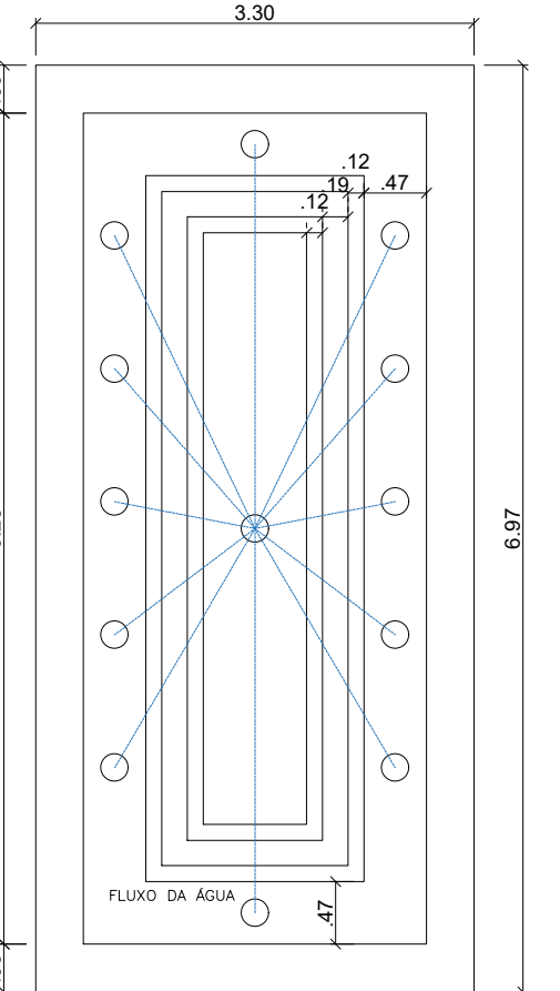
PLANTA PAGINAÇÃO - FONTE esc. 1:75
