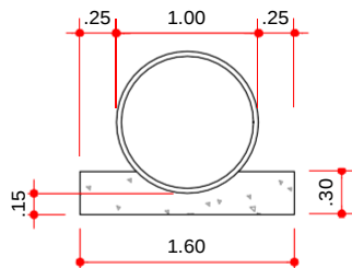
BERÇO EXTENSÃO=6,00m
