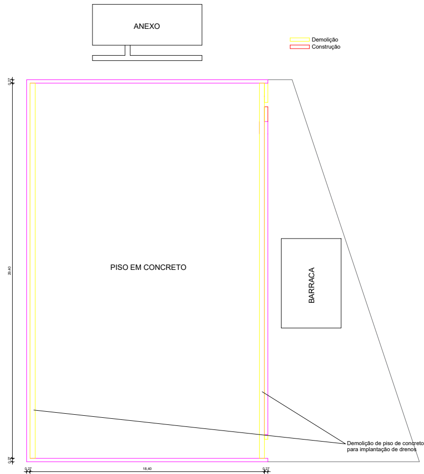
PLANTA BAIXA - DEMOLIÇÃO X CONSTRUÇÃO Escala ..... 1/100
