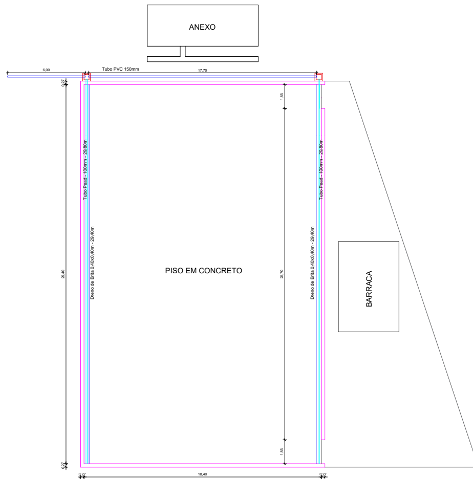
DRENAGEM Escala .....1/100
