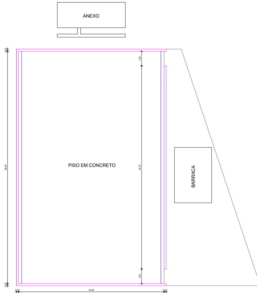
PLANTA BAIXA MODIFICADA Escala .....1/100
