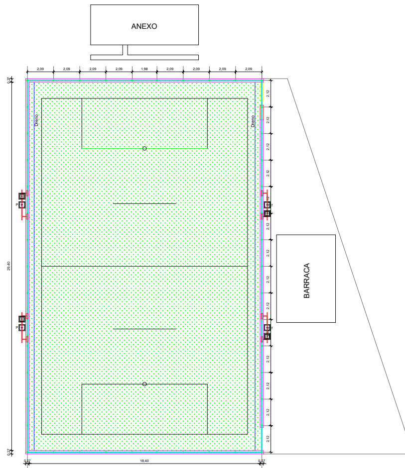
GRAMADO SINTÉTICO Escala .....1/100
