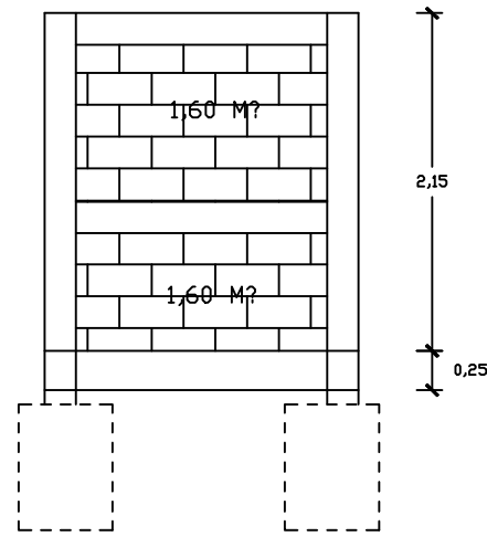
VISTA FRONTAL DA ALA 02 ESCALA = 1/50
