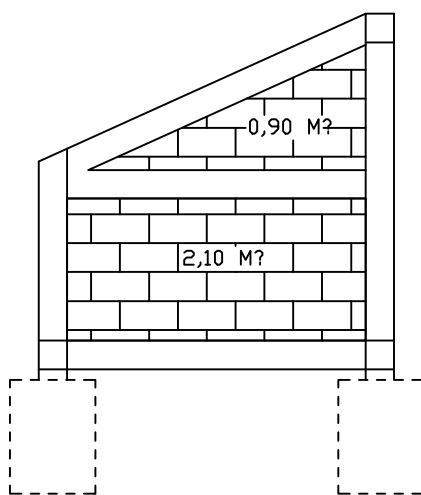
VISTA FRONTAL DA ALA 01 ESCALA = 1/50
