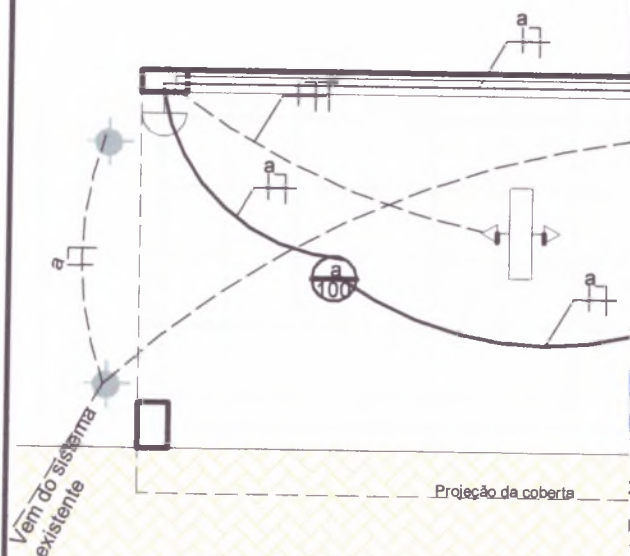
Planta de Coberta Escala: 1/100
