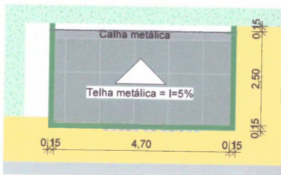
Planta de Coberta Escala: 1/100
