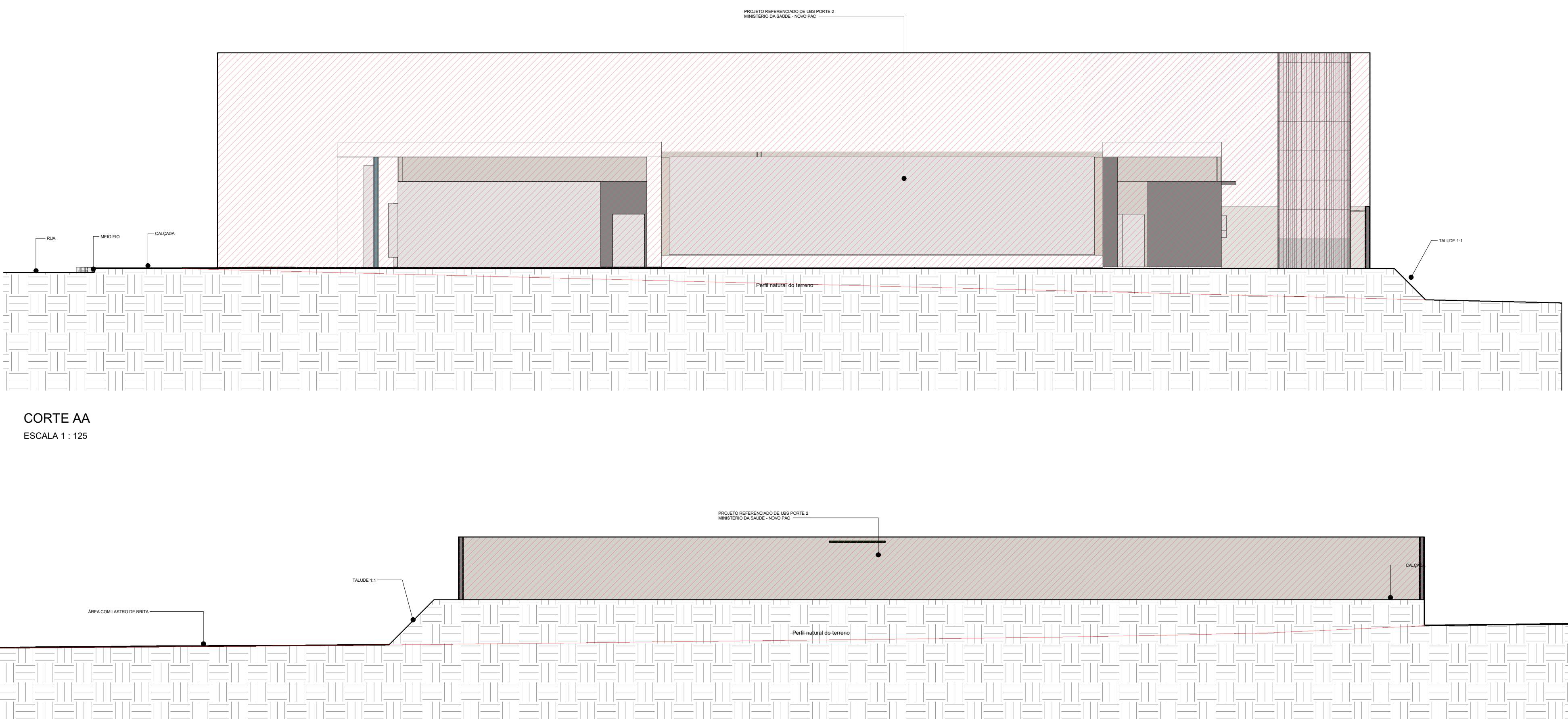
CORTE AA ESCALA 1 : 125 CORTE BB ESCALA 1 : 125
