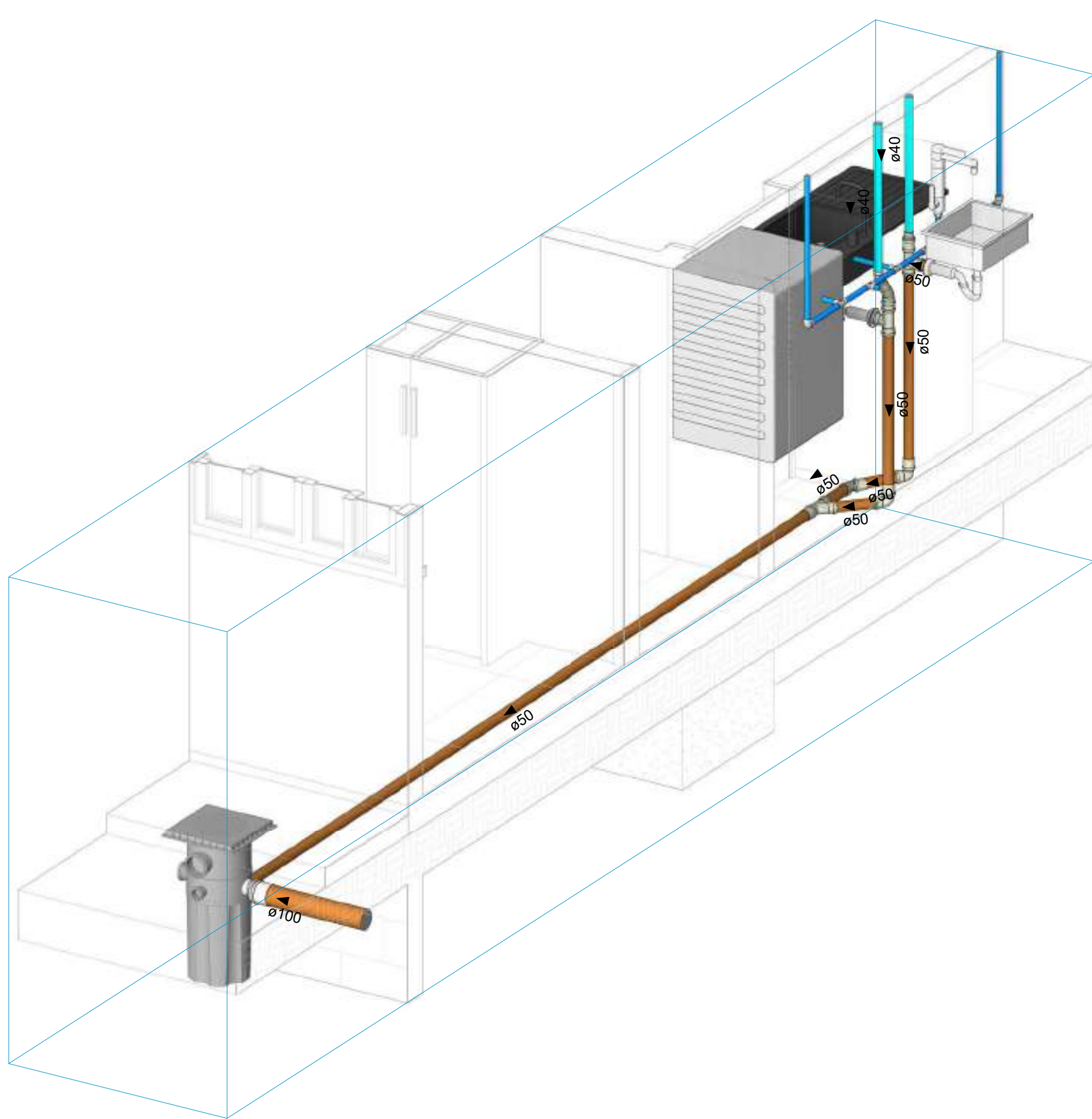
ISOMÉTRICO - COZINHA
