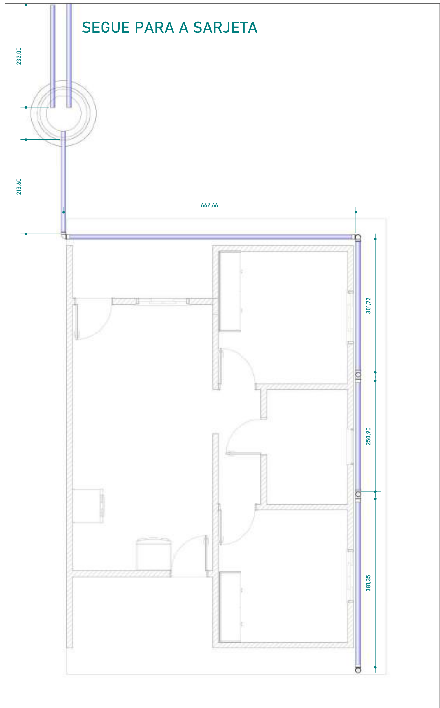
4 PLANTA BAIXA - ÁGUAS PLUVIAIS 1 : 50
