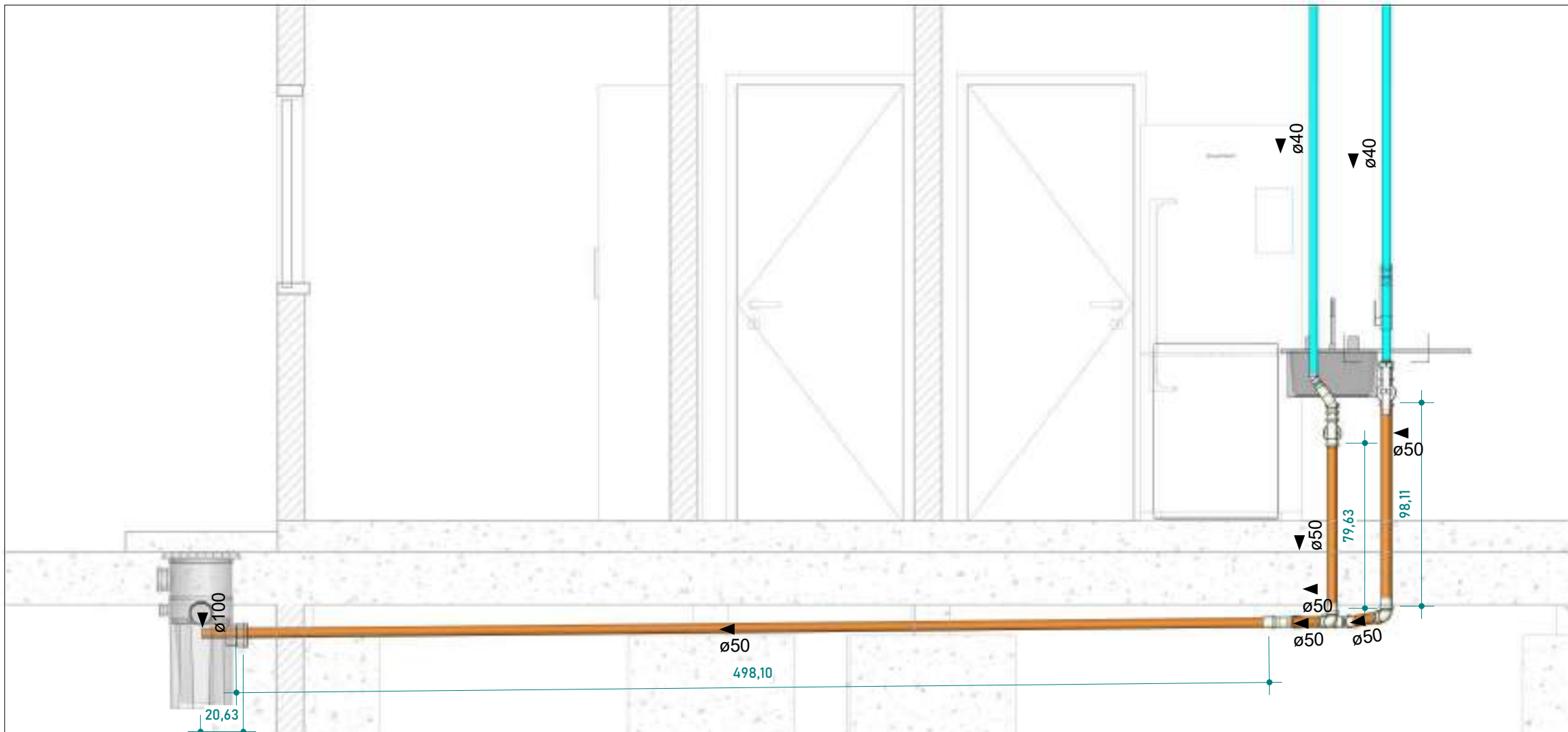
2 ELEVÇÃO - ESGOTO COZINHA 1 : 25
