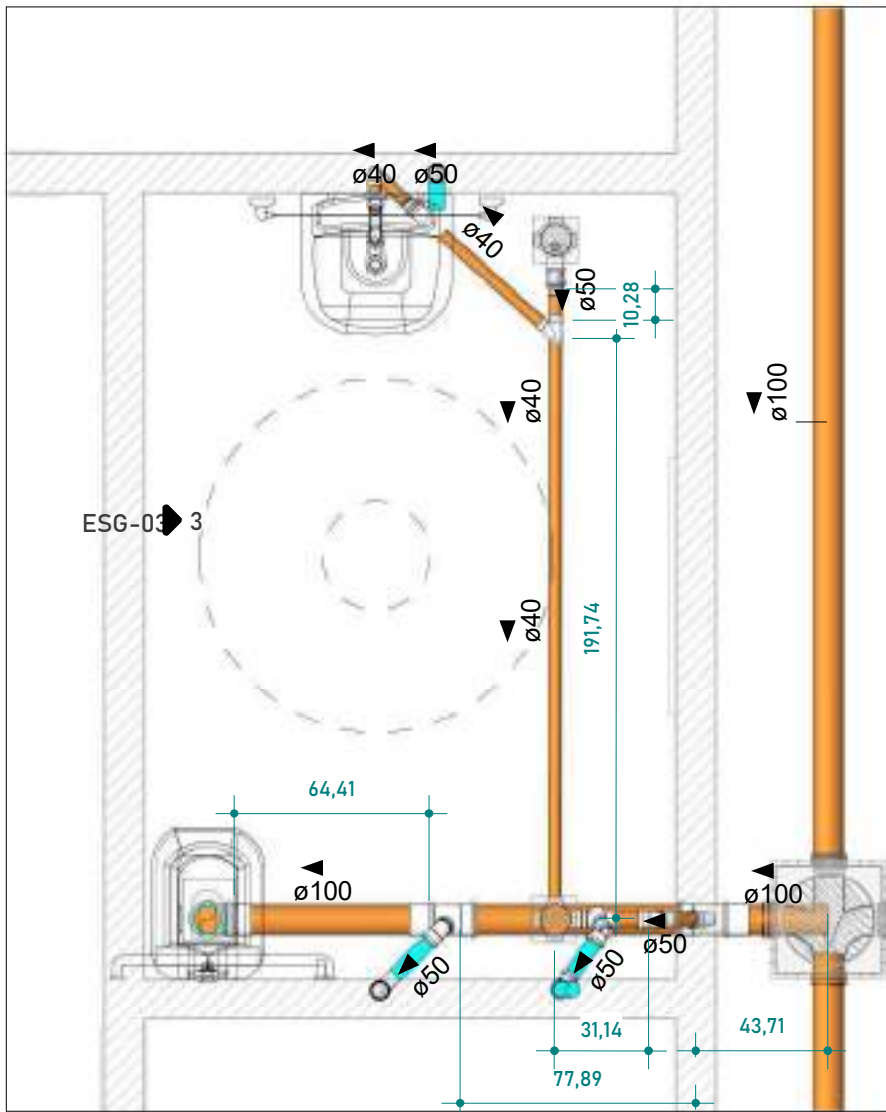
3 DETALHE - WC 1 : 25
