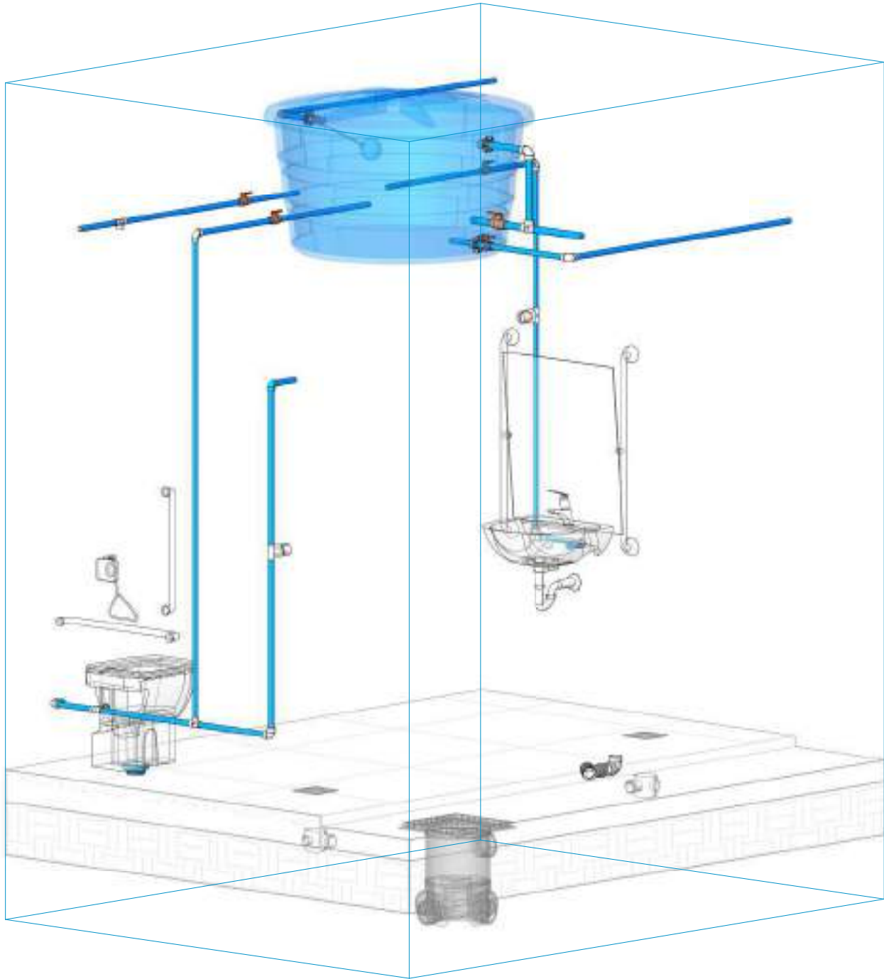
3D HID - Caixa Dagua
