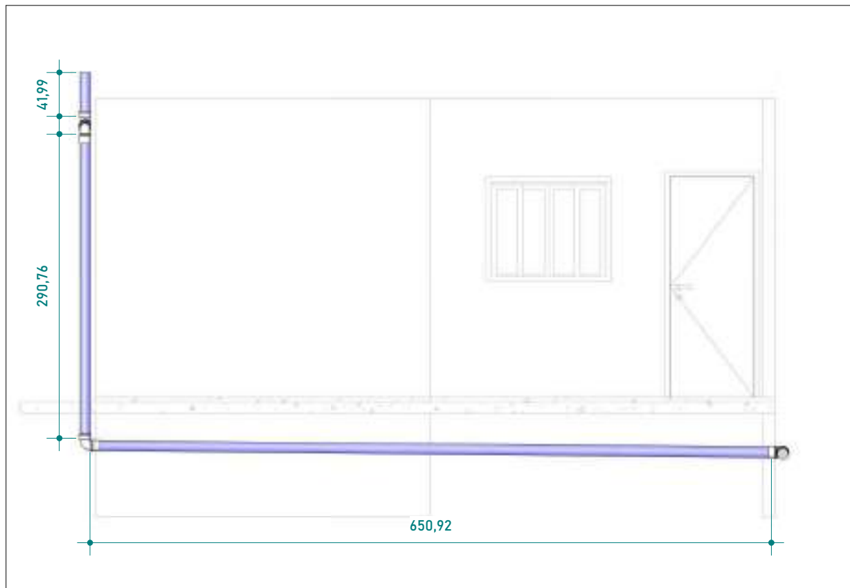
2 CORTE 002 1 : 50
