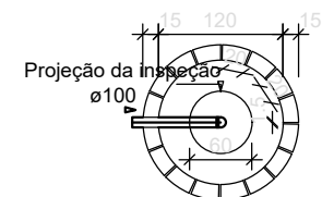
SUMIDOURO PLANTA BAIXA - ESC. 1:75
