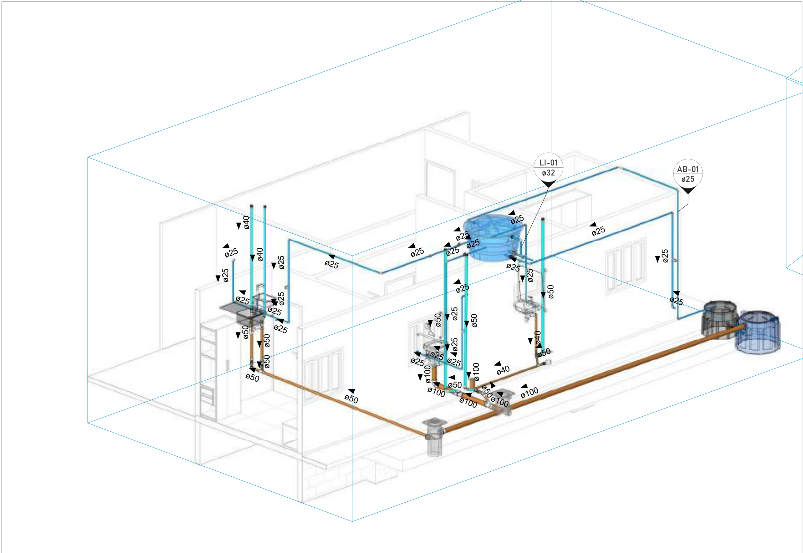
1 ISOMÉTRICO GERAL
