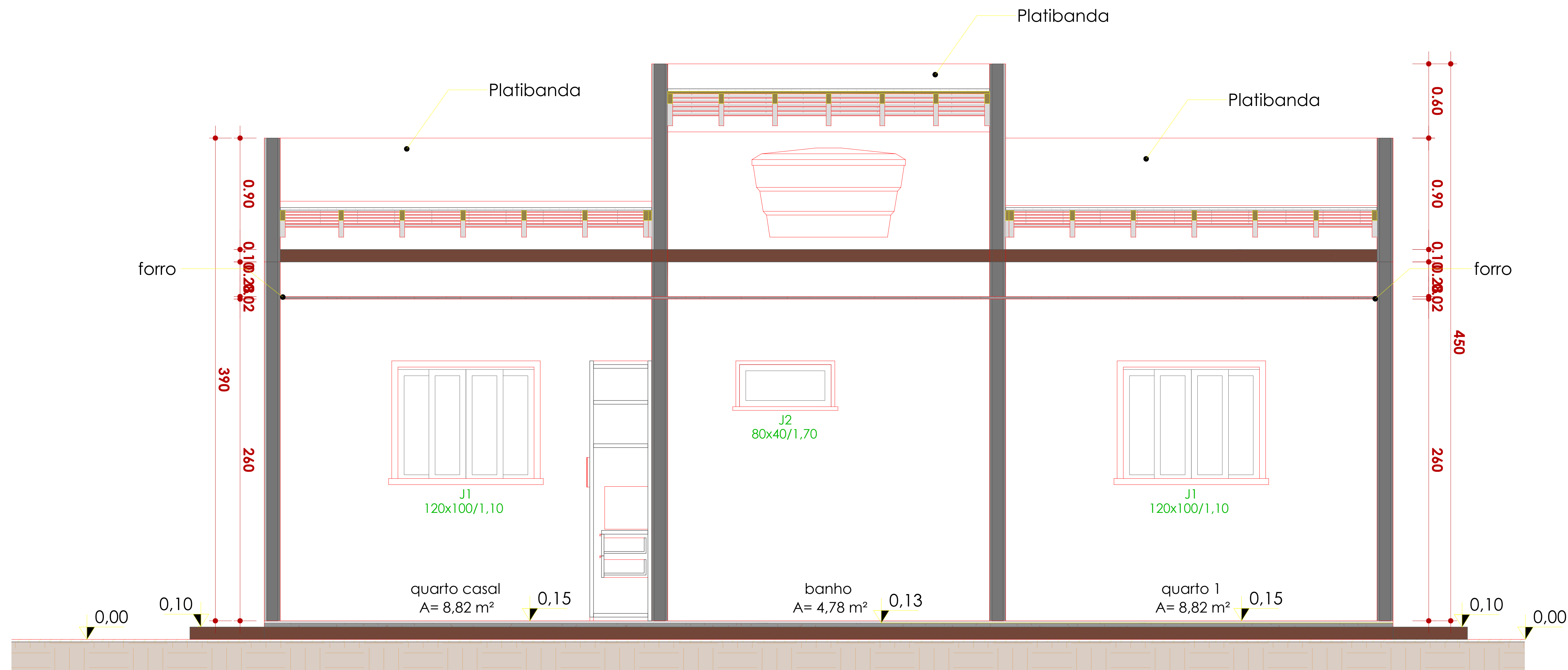
Corte BB esc.: 1:50
