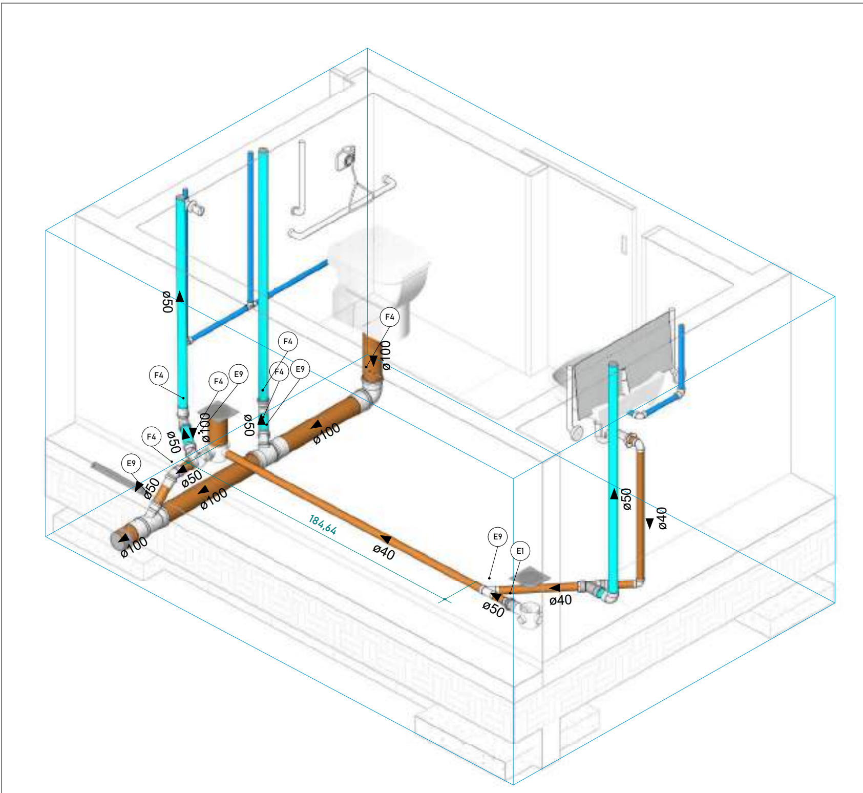
VISTA ISOMÉTRICA - WC
