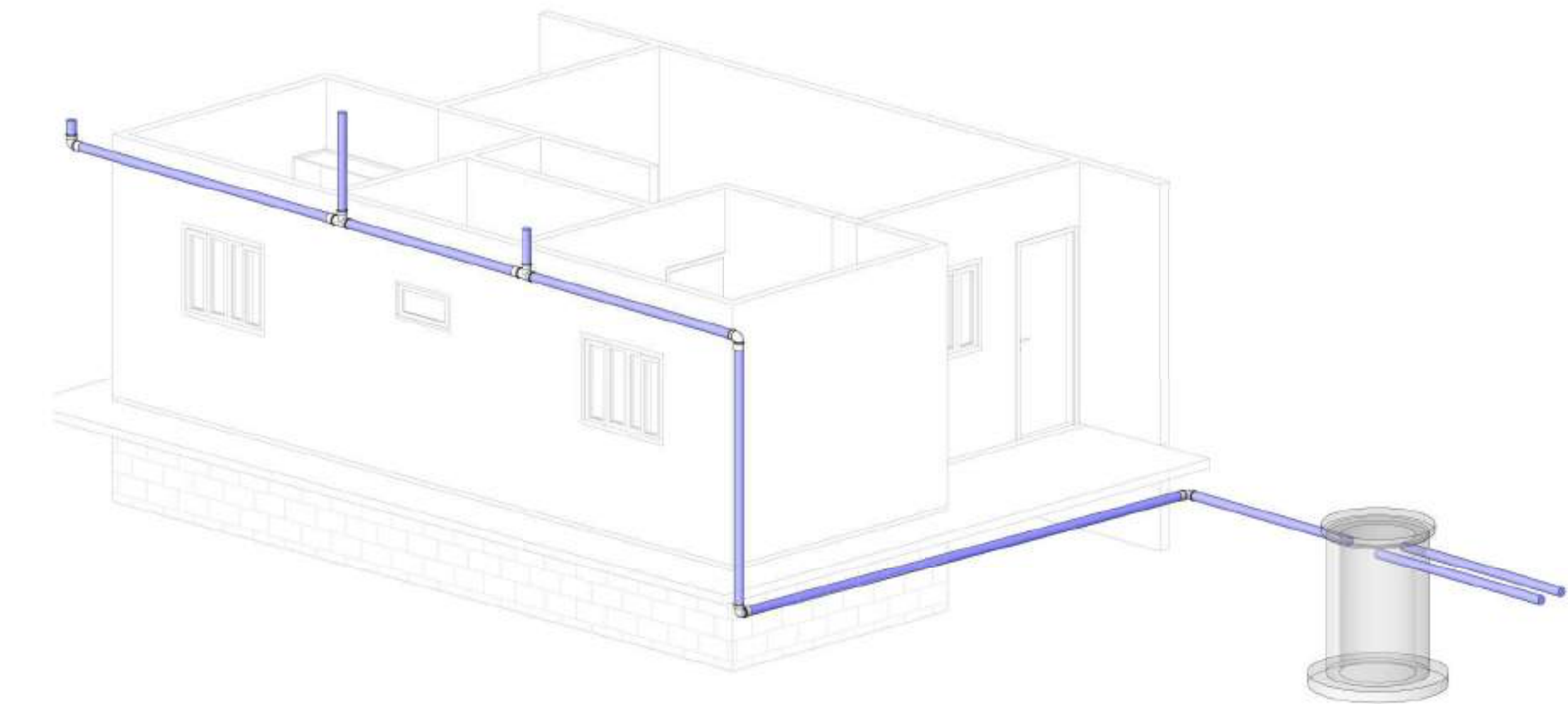
3 VISTA ISOMÉTRICA - ÁGUA PLUVIAL SIMPLES
