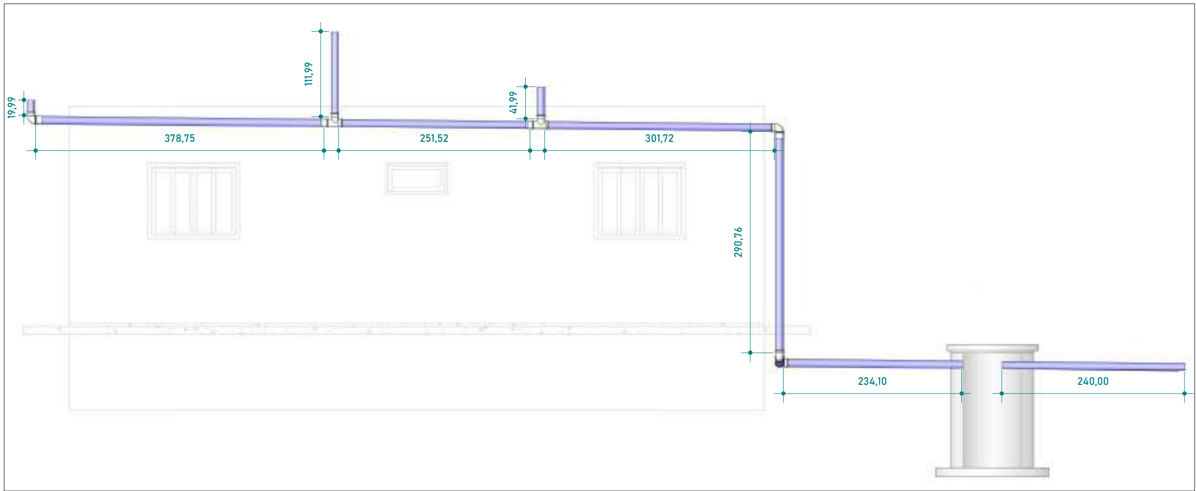
1 CORTE 001 1 : 50
