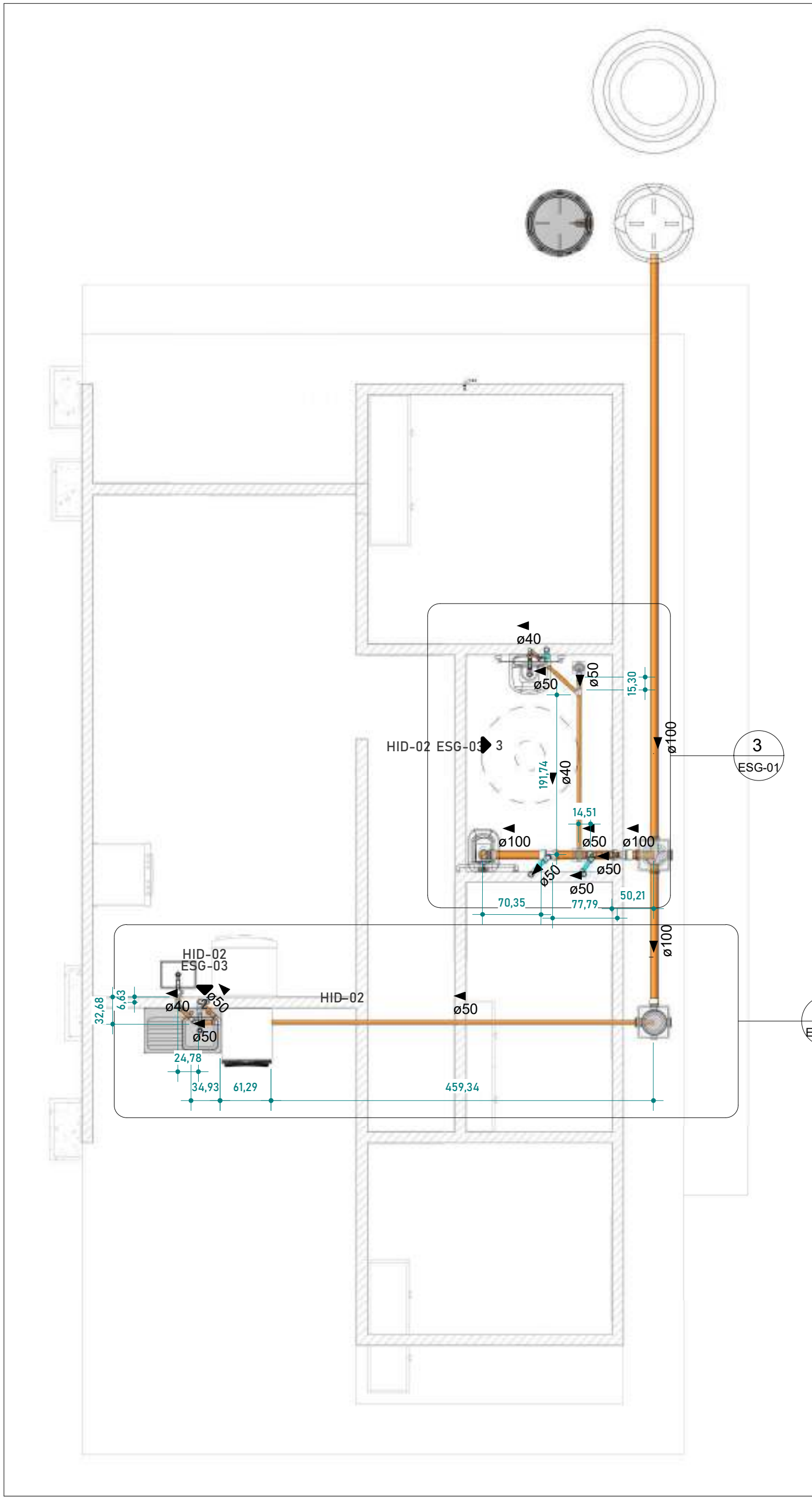
1 PLANTA ESG 1 : 50
